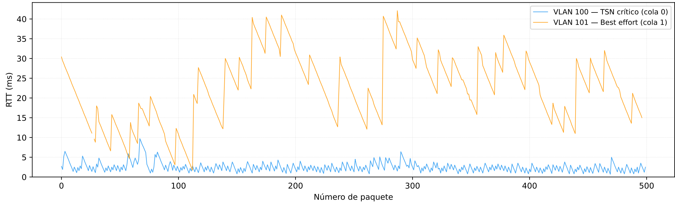
Latencia RTT medida — cadena BR1→BR2→BR3
