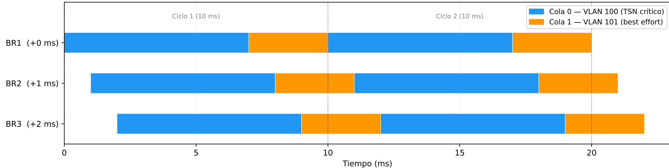
Diagrama de tiempo TAS teórico — cadena BR1→BR2→BR3
