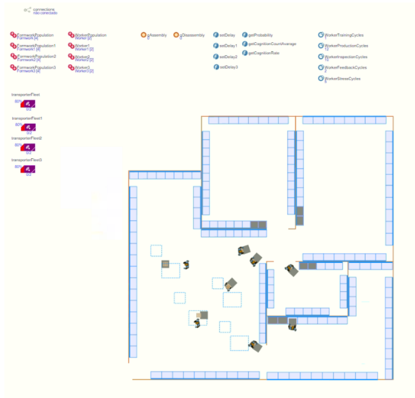
Figura 45 – Visualização da simulação em 2D no AnyLogic.
