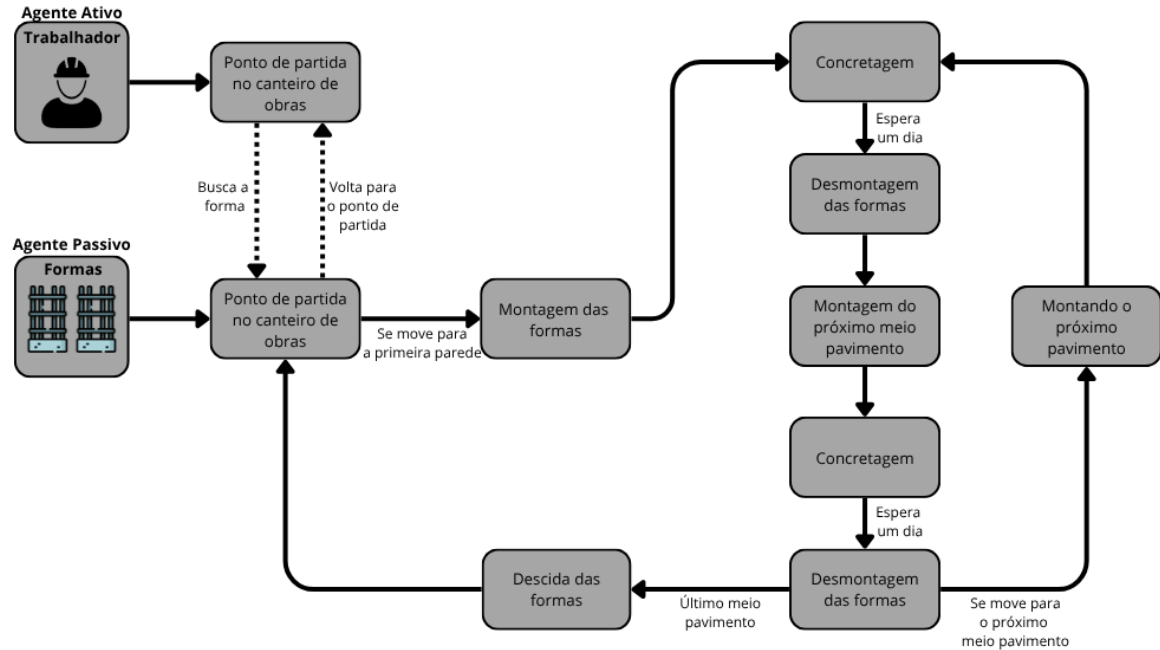
Figura 10 – Etapas gerais do processo de produção de paredes de concreto em um edifício.
