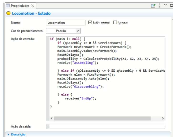
Figura 40 – Lógica do estado Locomotion .
