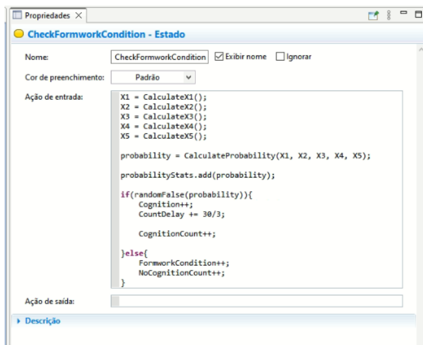
Figura 42 – Exemplo de lógica aplicada às atividades.
