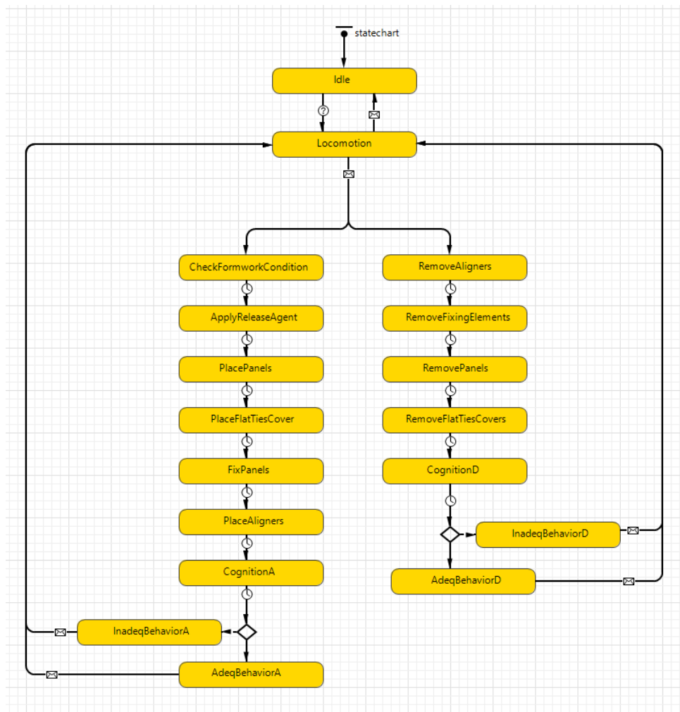
Figura 32 – Diagrama de Estados na ABM.
