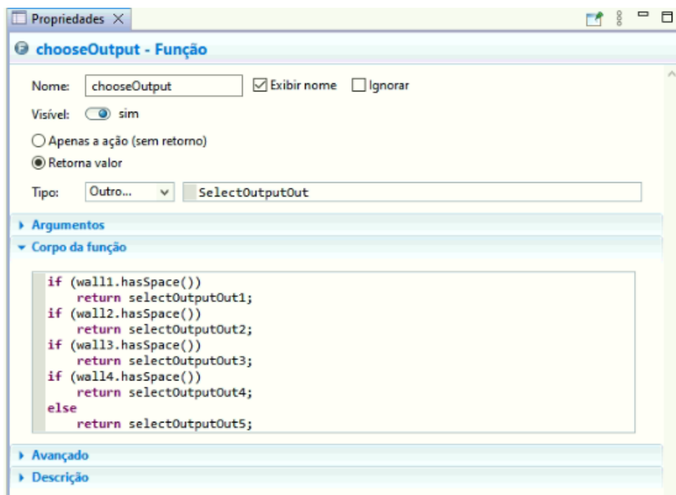
Figura 26 – Propriedades lógicas da função chooseOutput .
