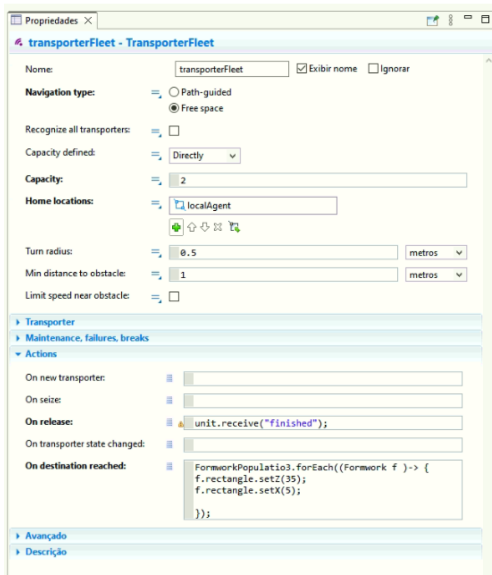
Figura 24 – Propriedades do Transporter Fleet com movimentação livre.
