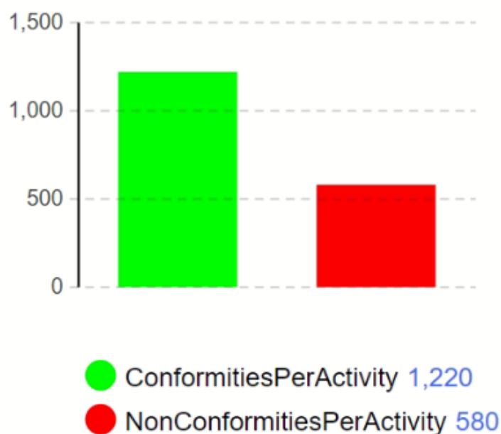
Figura 52 – Resultado das conformidades por atividade com todos os fatores de influência no valor mínimo (1).
