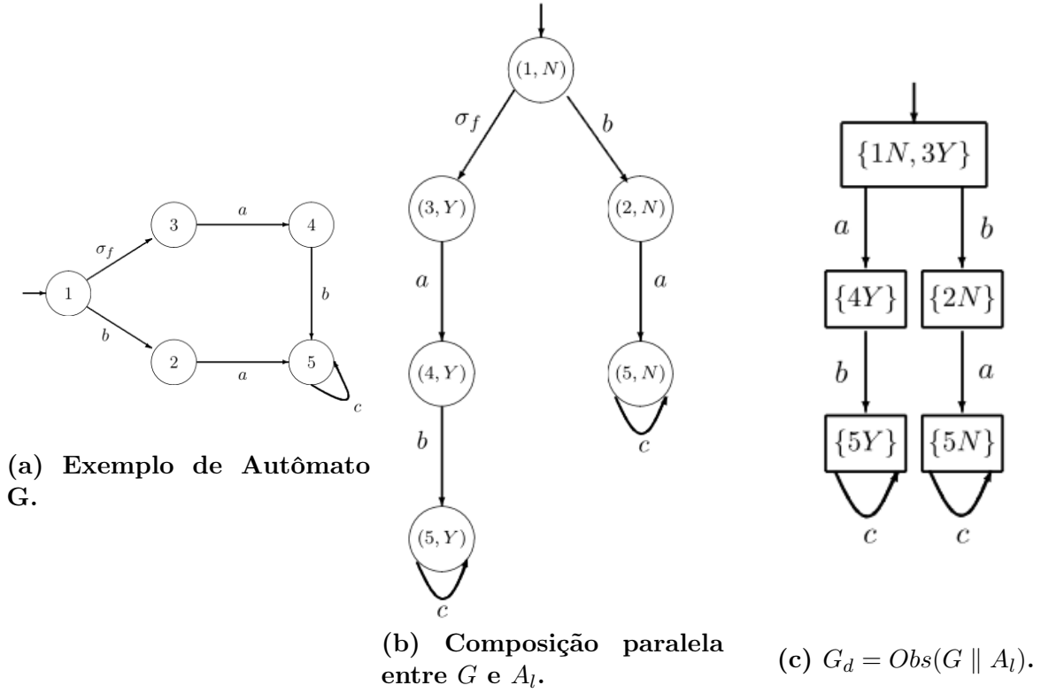
Figura 8 – Exemplo de construção de um autômato diagnosticador G_d .
