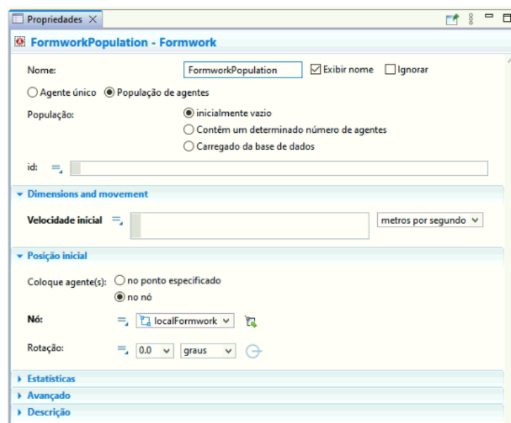
Figura 20 – Propriedades da população de fôrmas.
