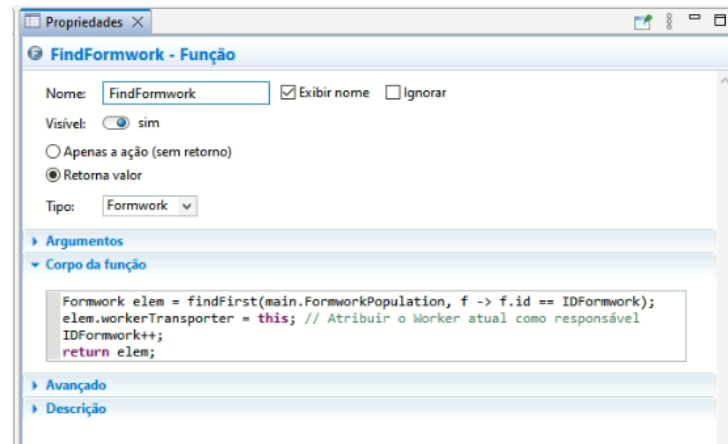
Figura 41 – Função FindFormwork para auxiliar na desmontagem.
