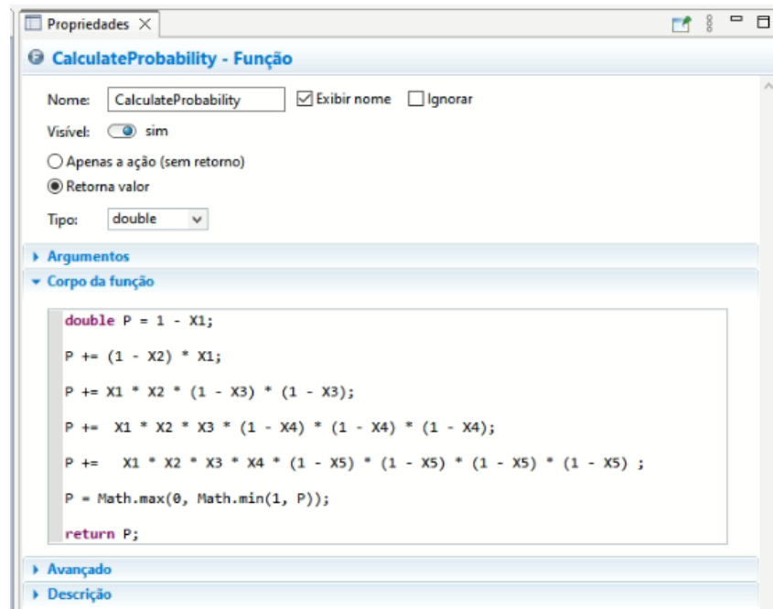
Figura 43 – Função para cálculo da probabilidade de pular a etapa.
