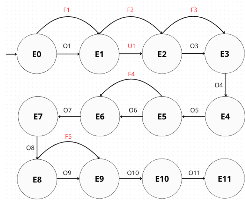
Figura 50 – Autômato gerador G do sistema.
