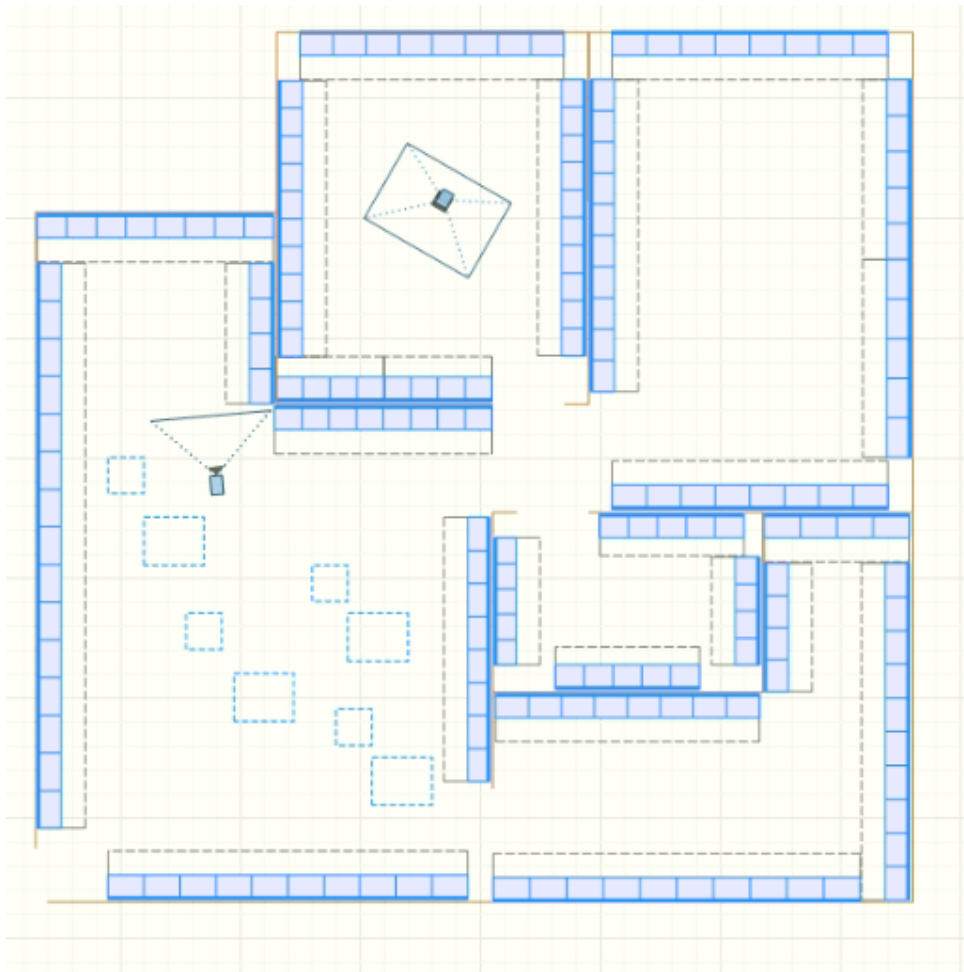
Figura 23 – Representação geométrica do cômodo e blocos no ambiente do AnyLogic.
