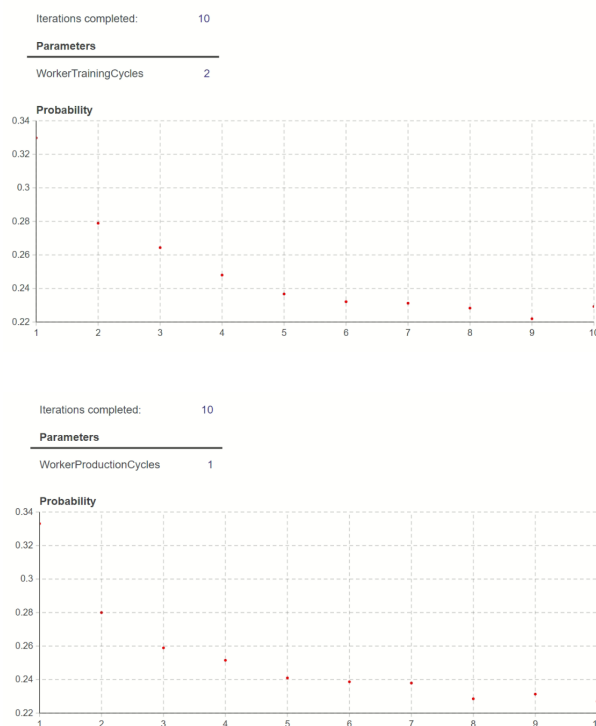
Figura 58 – Resultados da Sensitivity Analysis para os cenários analisados.
