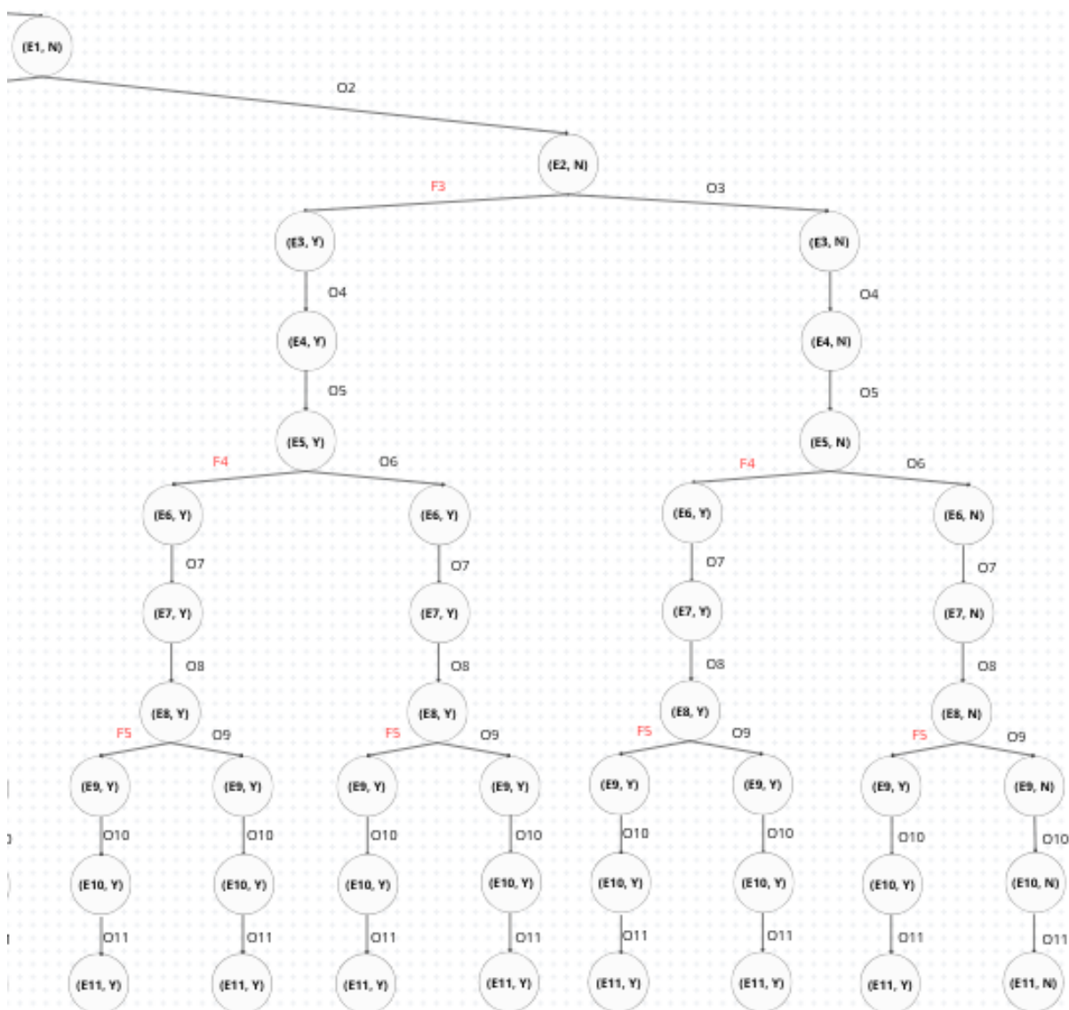
Figura 65 – Resultado da composição paralela do cenário modificado (Parte 4).
