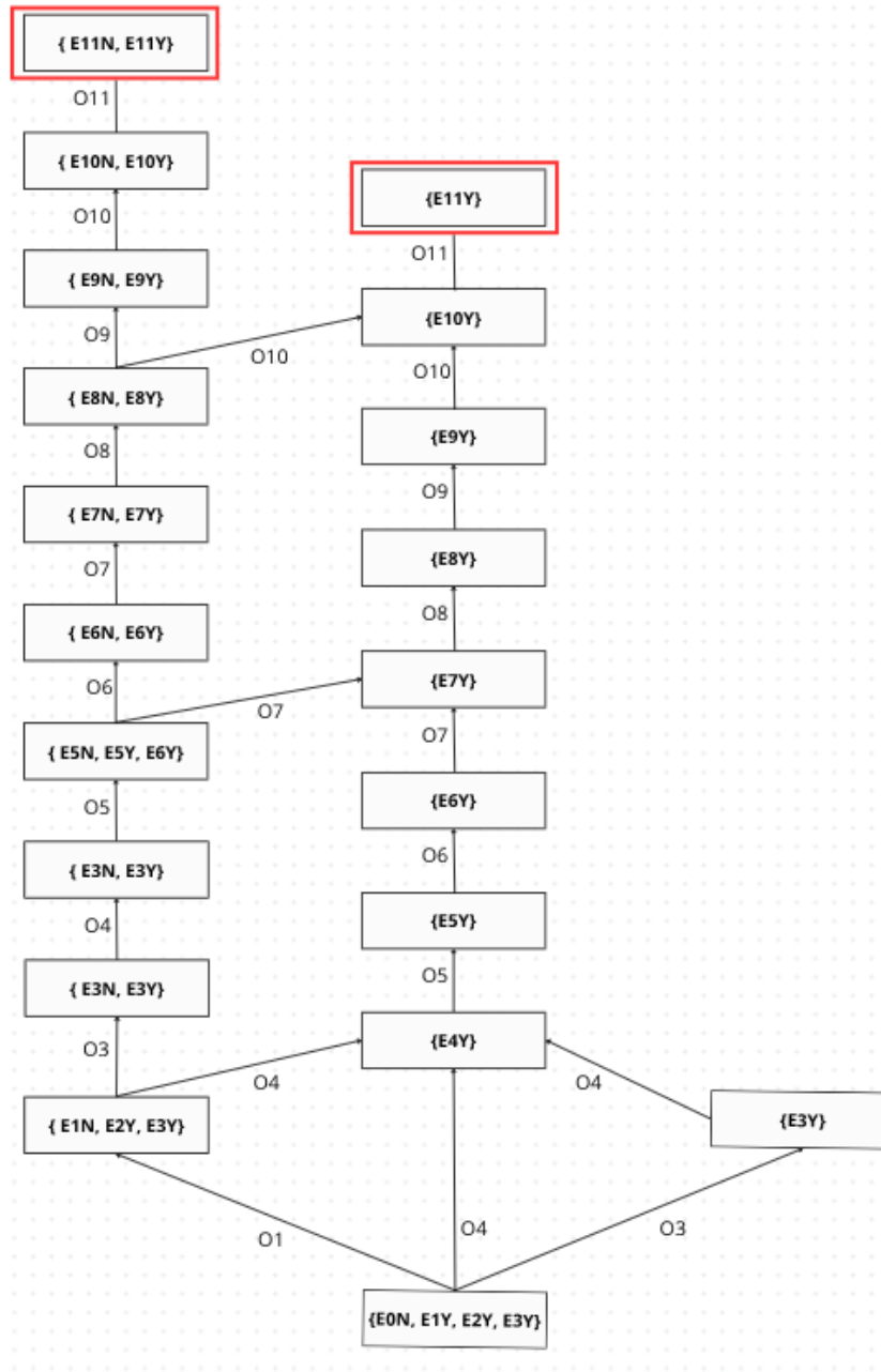
Figura 62 – Estados finais do Autômato Diagnosticador.
