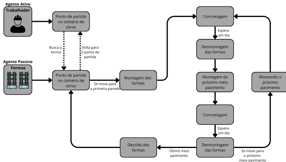
Figura 10 – Etapas gerais do processo de produção de paredes de concreto em um edifício.
