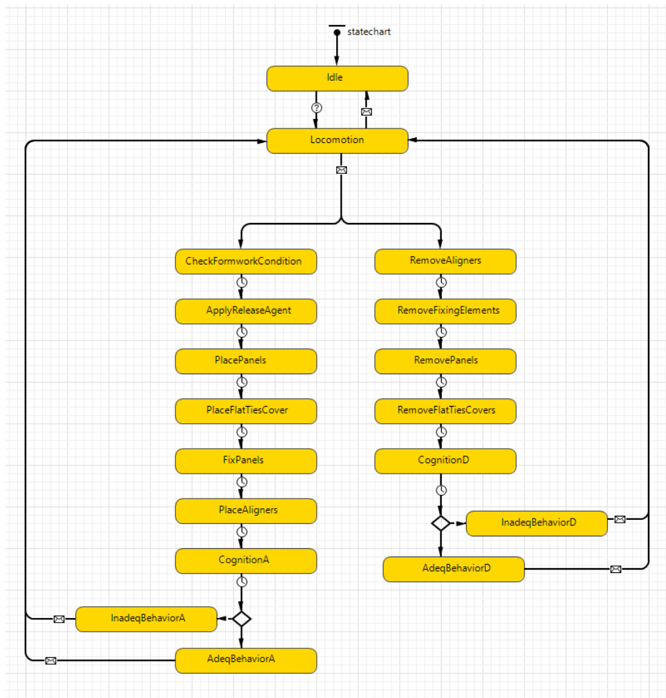
Figura 30 – Diagrama de estados na ABM.
