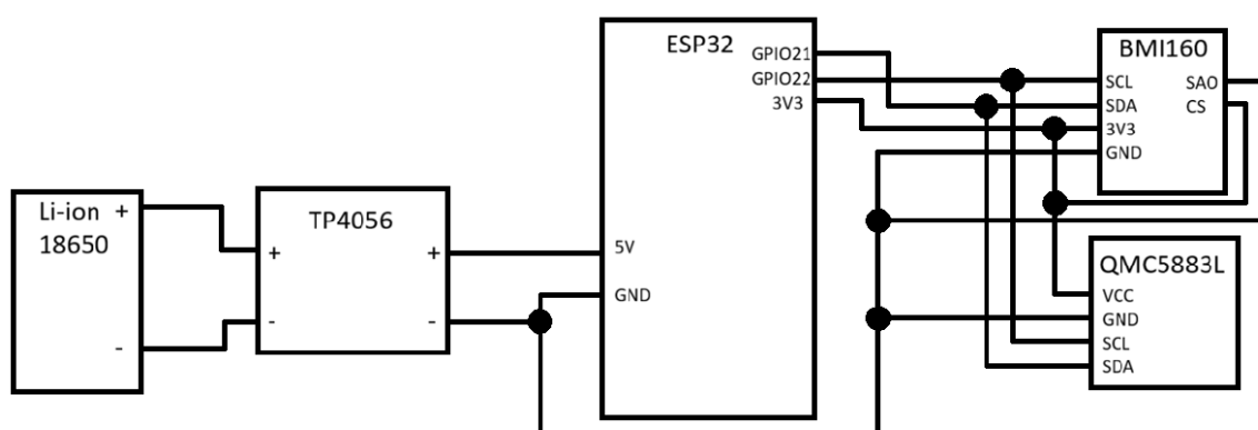
Obrázek 2: Blokové Schéma
