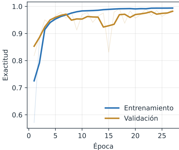
Exactitud
