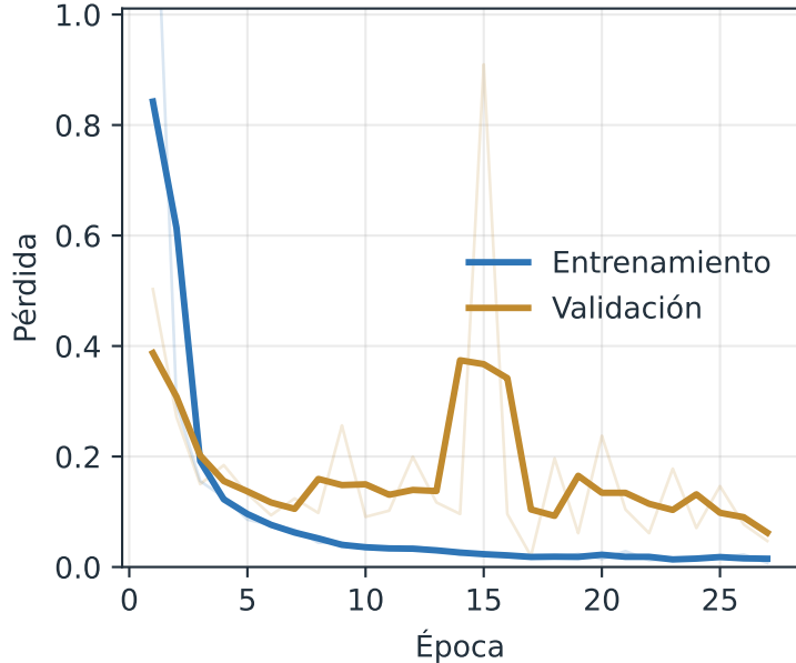
Pérdida
