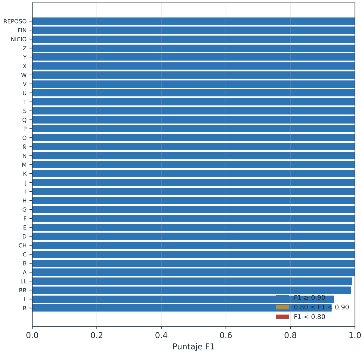
Puntaje F1 por clase (Modelo A)
