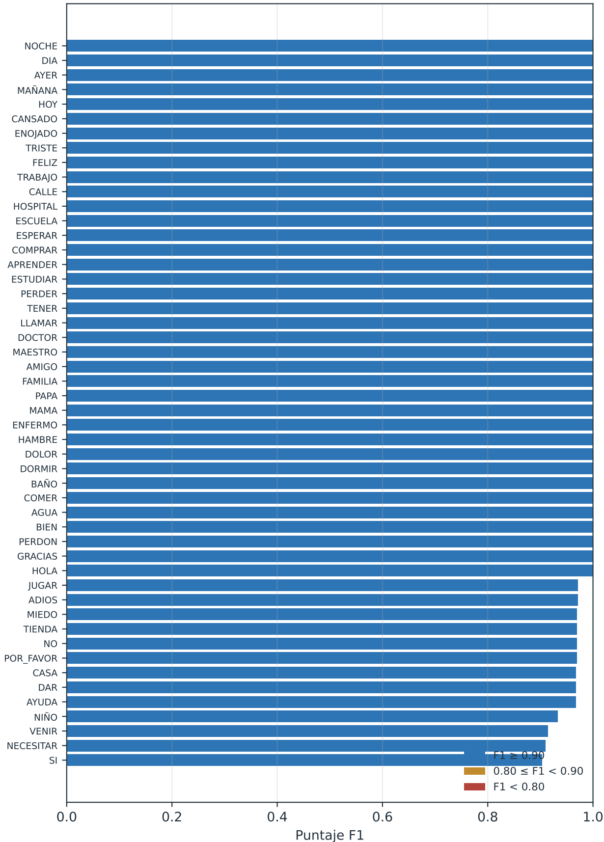
Puntaje F1 por clase (Modelo B)
