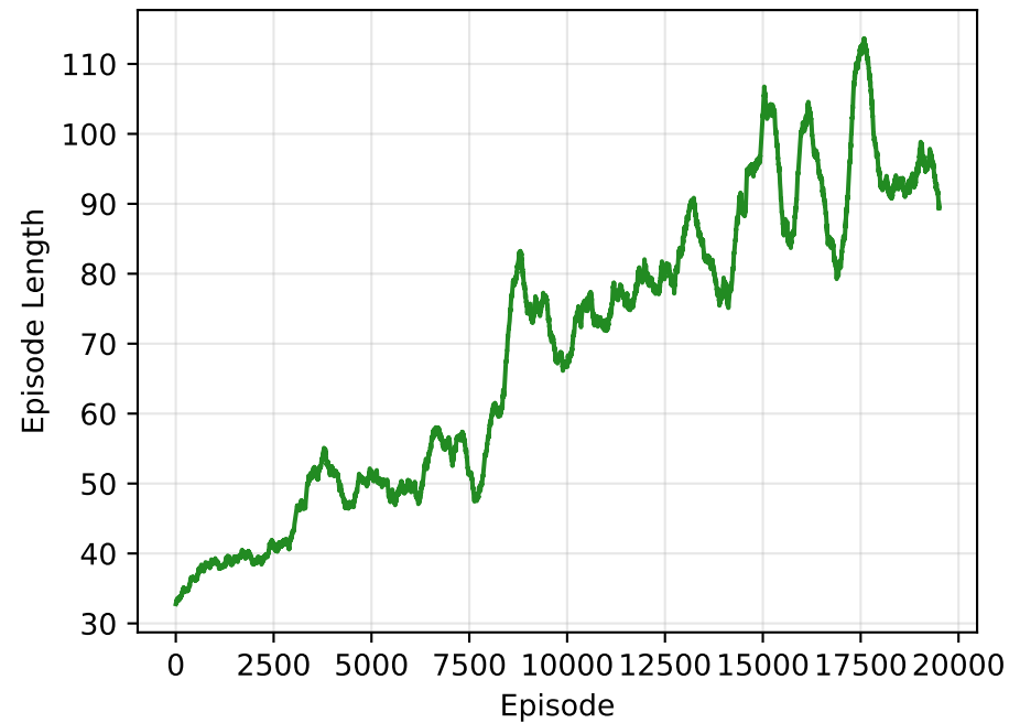
DQN — 8x8 Slippery
