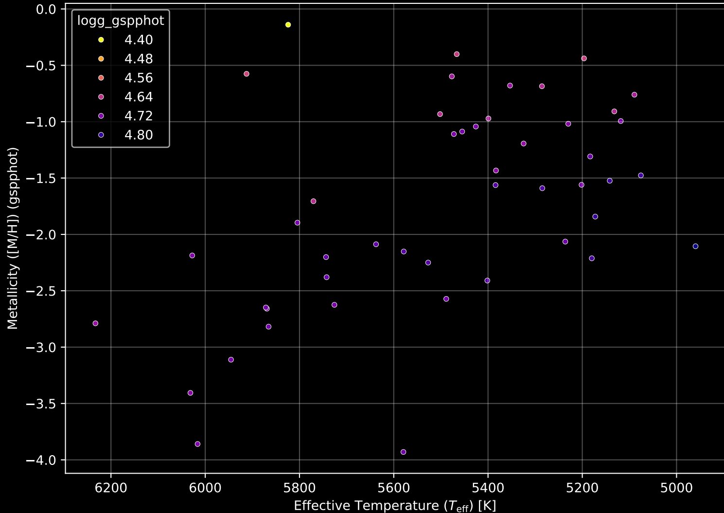
Gaia Stream: [C-11] Stellar Population Parameters (n= 47)
