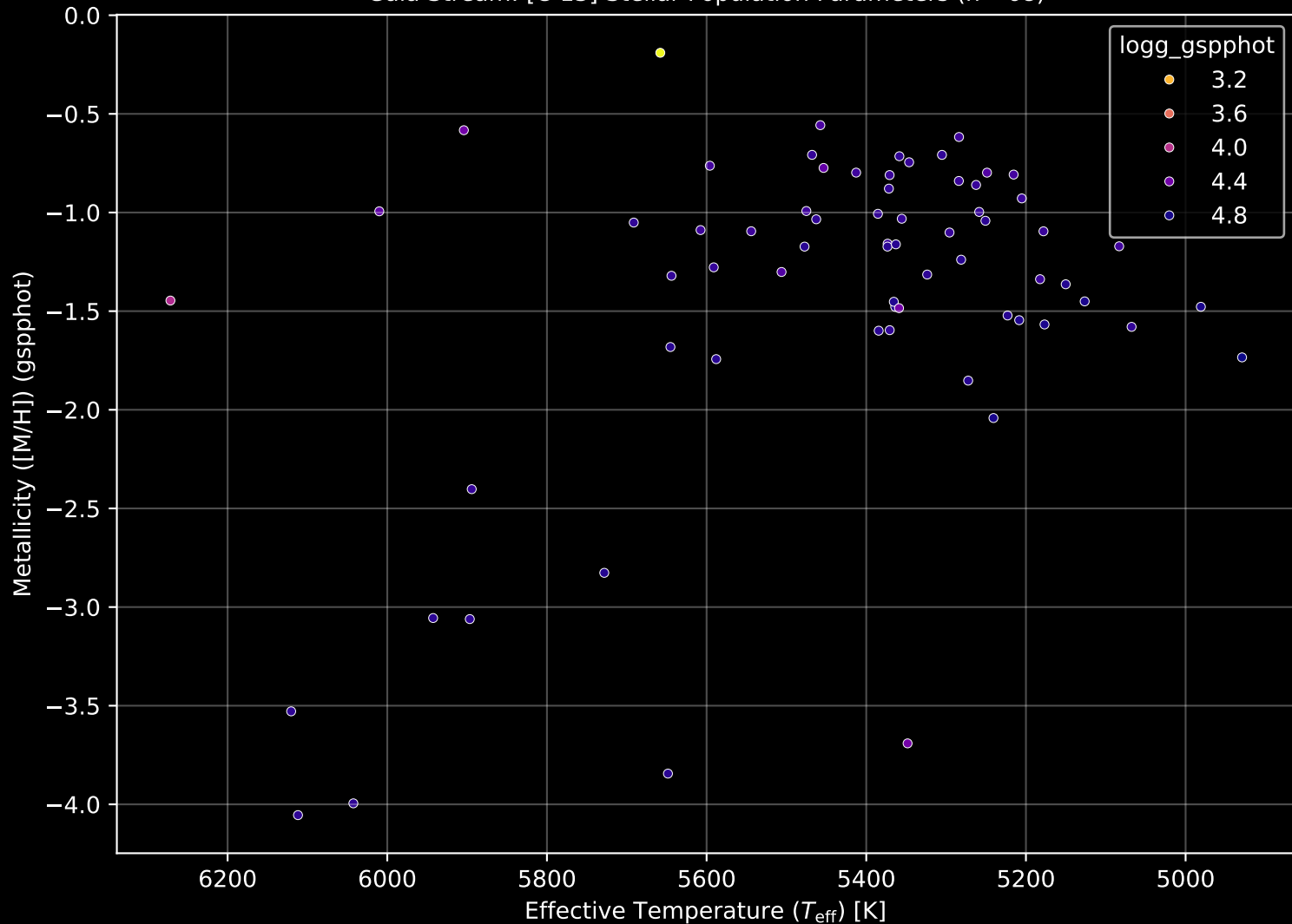
Gaia Stream: [C-13] Stellar Population Parameters (n= 68)
