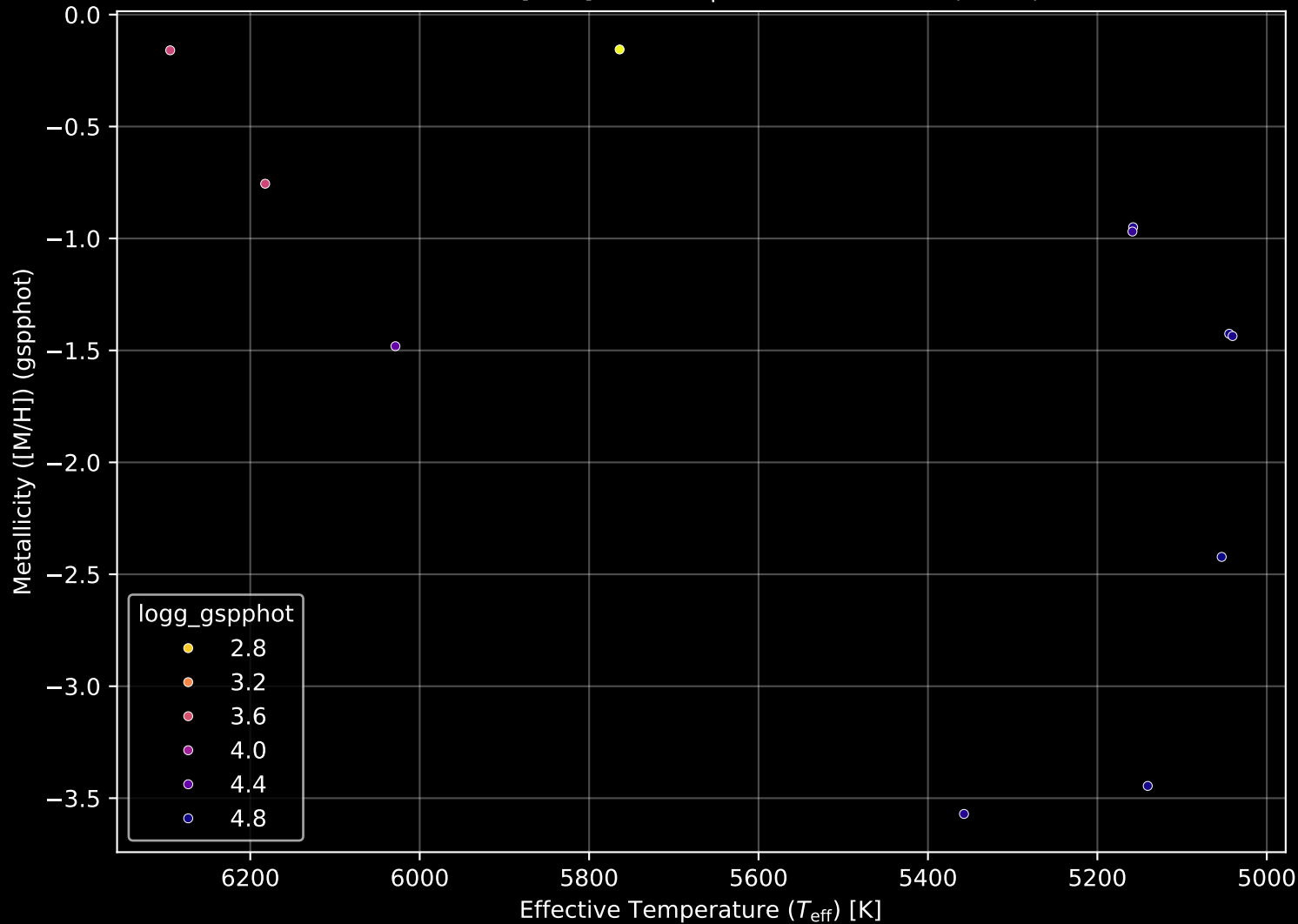
Gaia Stream: [C-19] Stellar Population Parameters (n= 11)
