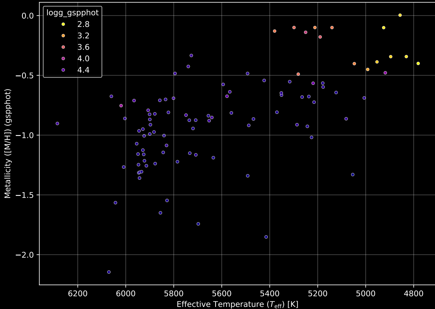
Gaia Stream: [C-24] Stellar Population Parameters (n= 97)
