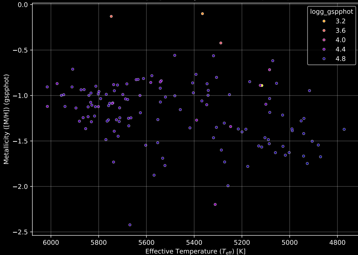
Gaia Stream: [C-9] Stellar Population Parameters (n= 134)
