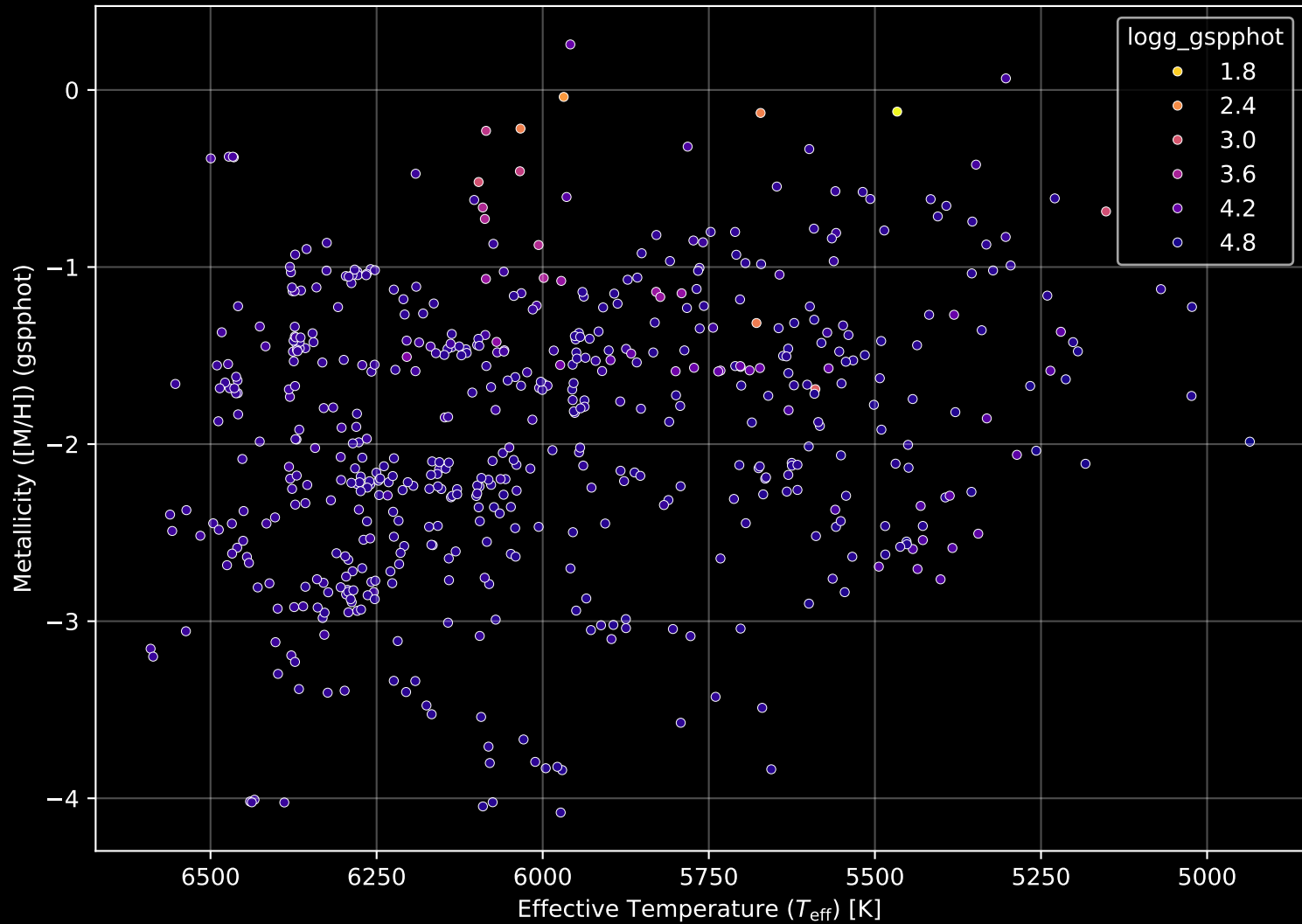
Gaia Stream: [GD-1] Stellar Population Parameters (n= 555)
