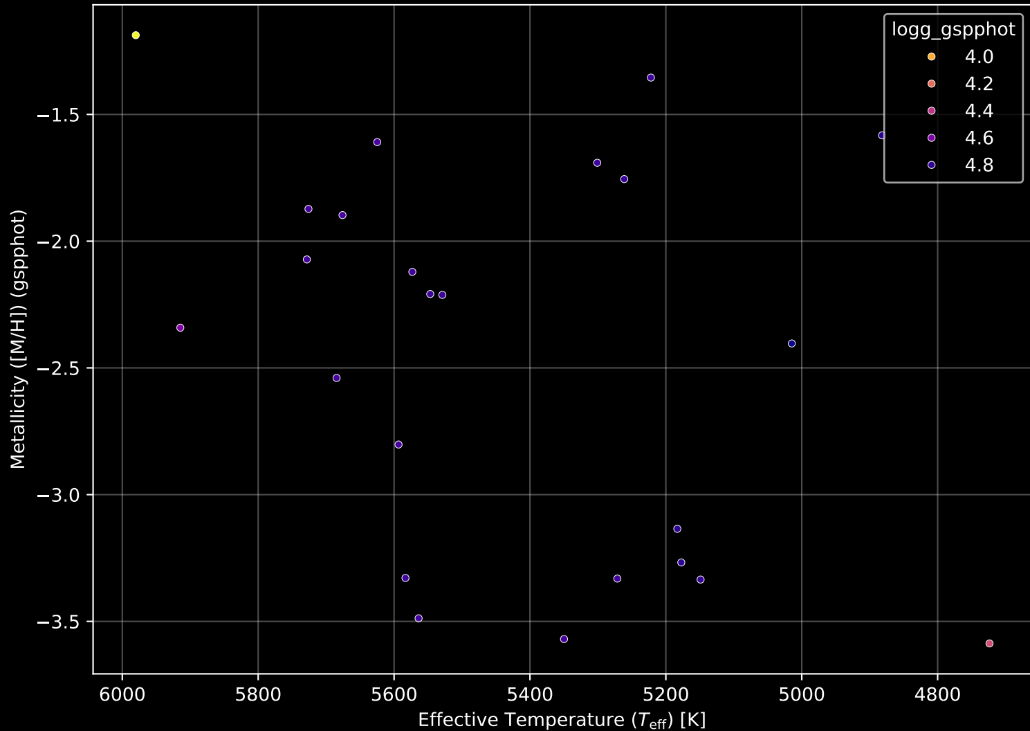
Gaia Stream: [Gaia-12] Stellar Population Parameters (n= 24)
