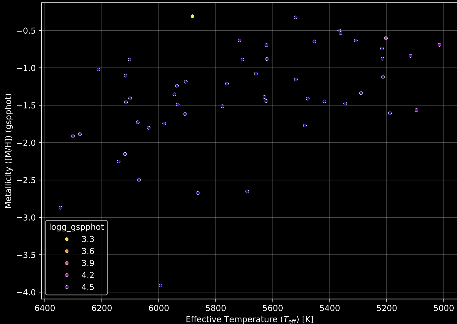
Gaia Stream: [Gaia-6] Stellar Population Parameters (n= 51)
