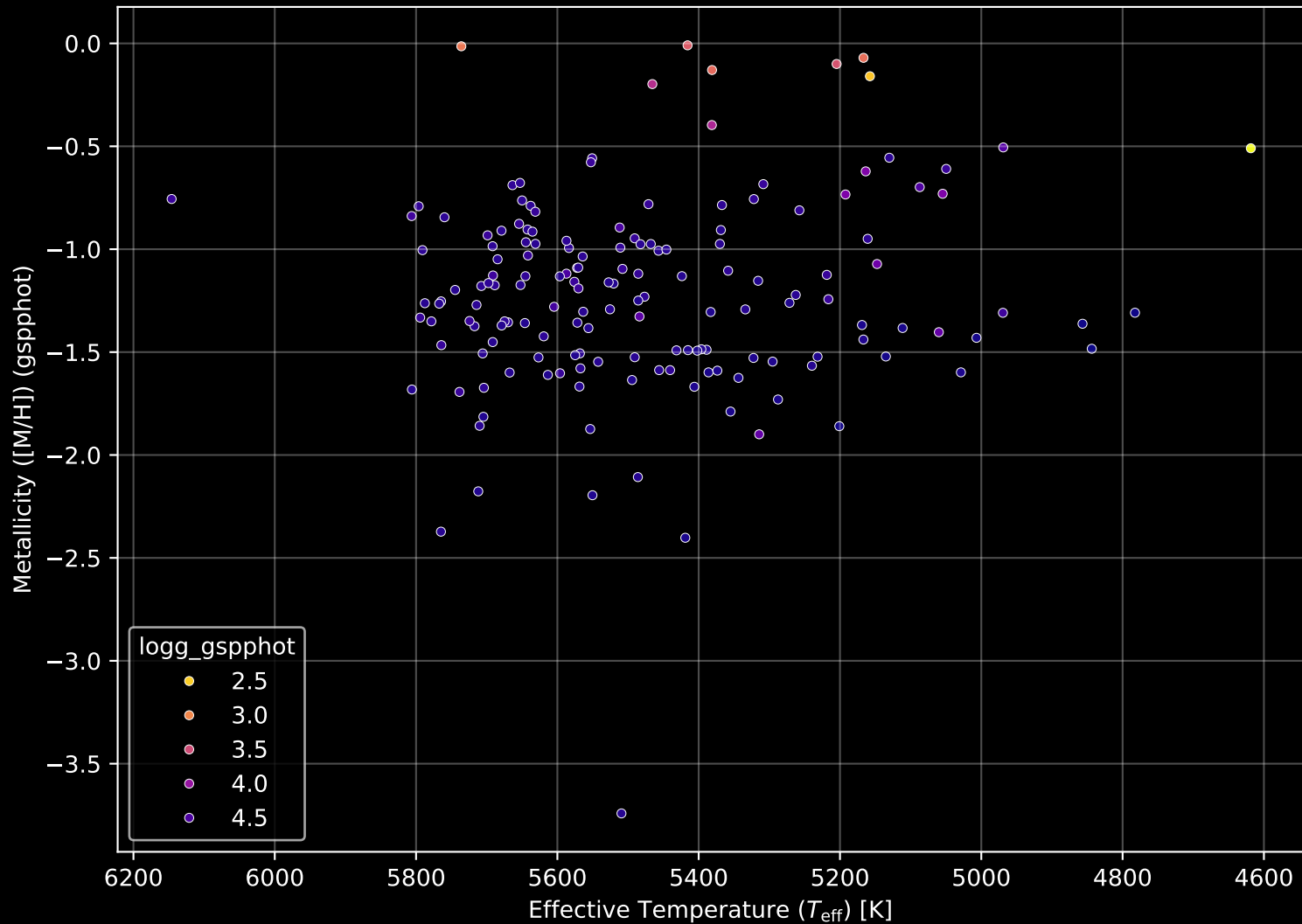
Gaia Stream: [Gaia-7] Stellar Population Parameters (n= 160)
