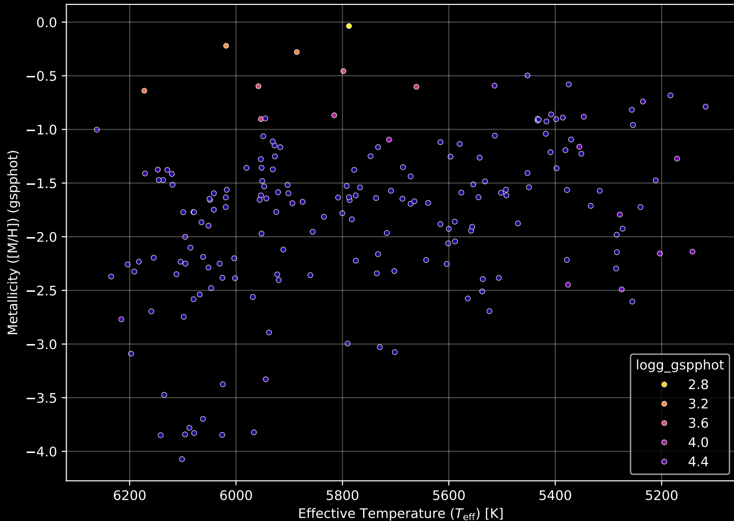
Gaia Stream: [Gaia-8] Stellar Population Parameters (n= 191)
