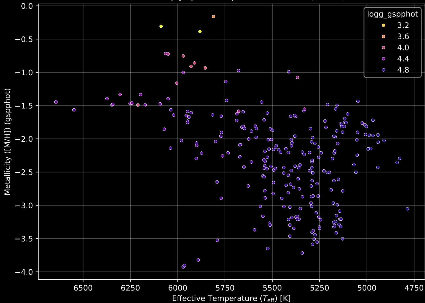
Gaia Stream: [Gjoll] Stellar Population Parameters (n= 249)
