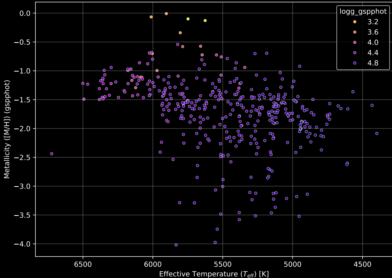
Gaia Stream: [Hrid] Stellar Population Parameters (n= 393)
