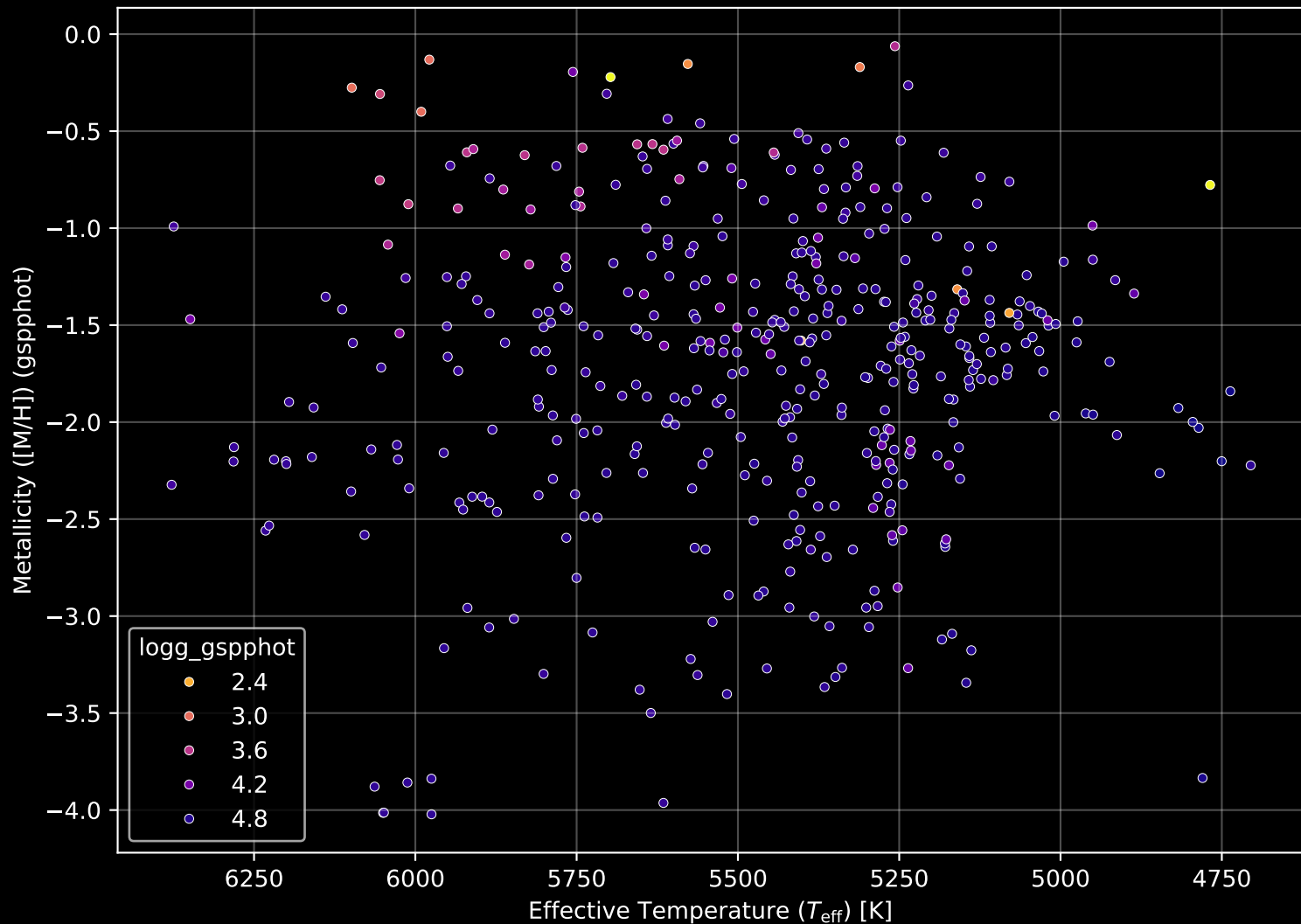
Gaia Stream: [Indus] Stellar Population Parameters (n= 442)
