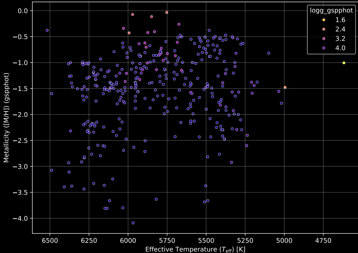
Gaia Stream: [Jhelum] Stellar Population Parameters (n= 350)
