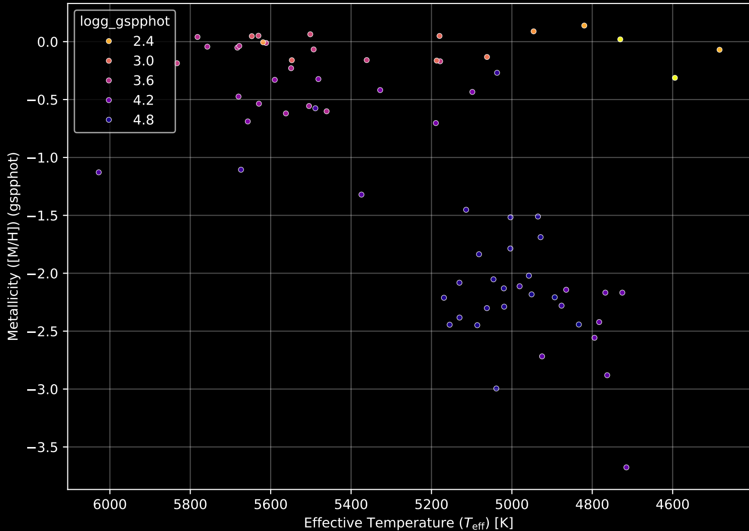
Gaia Stream: [Kwando] Stellar Population Parameters (n= 69)
