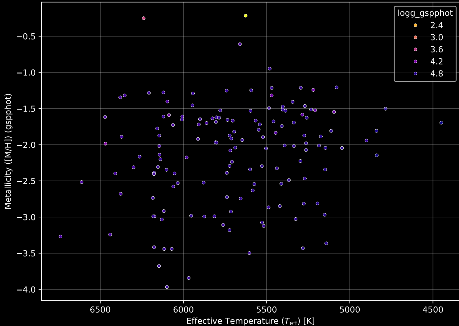
Gaia Stream: [Leiptr] Stellar Population Parameters (n= 145)
