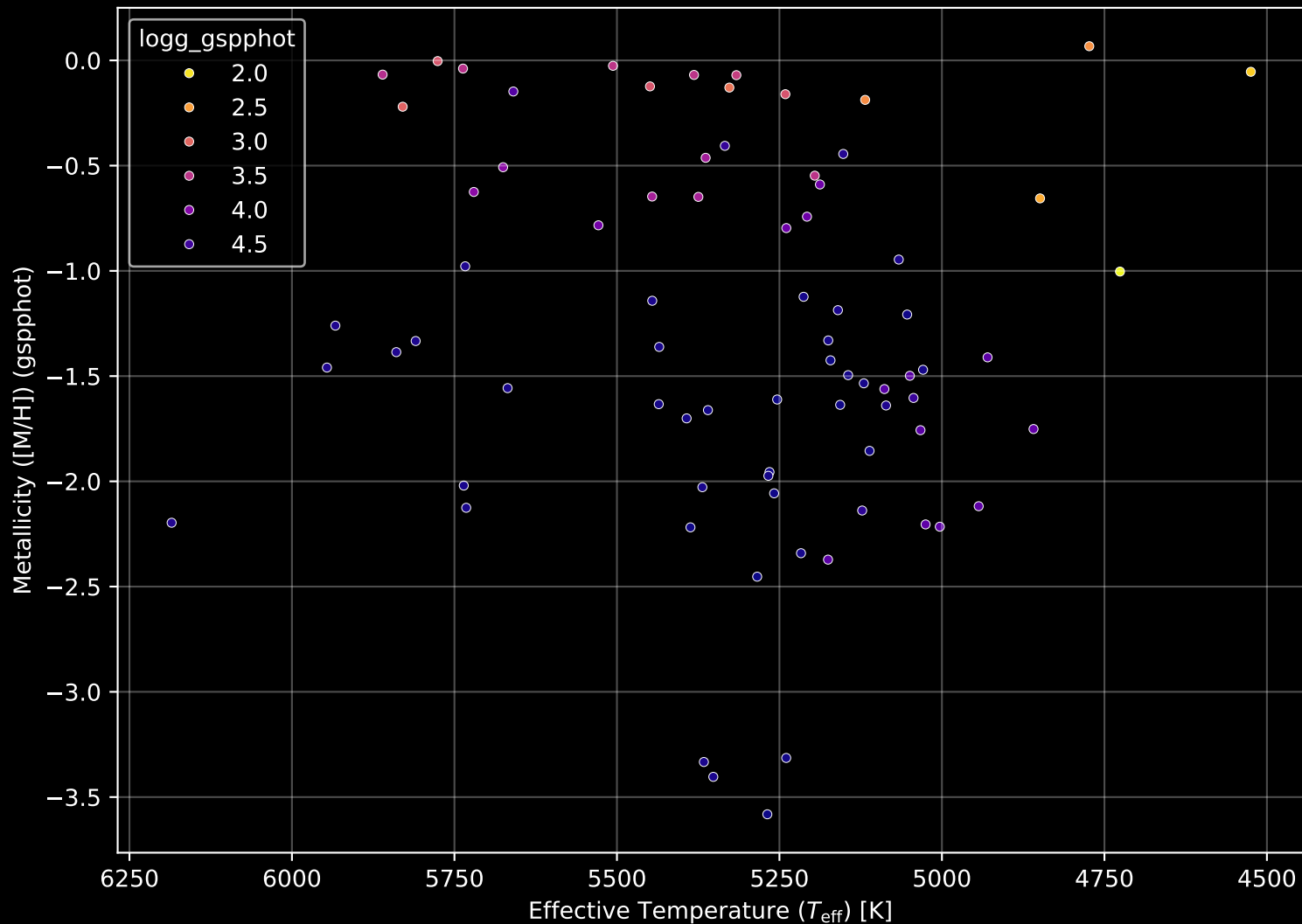
Gaia Stream: [NGC1261] Stellar Population Parameters (n= 77)
