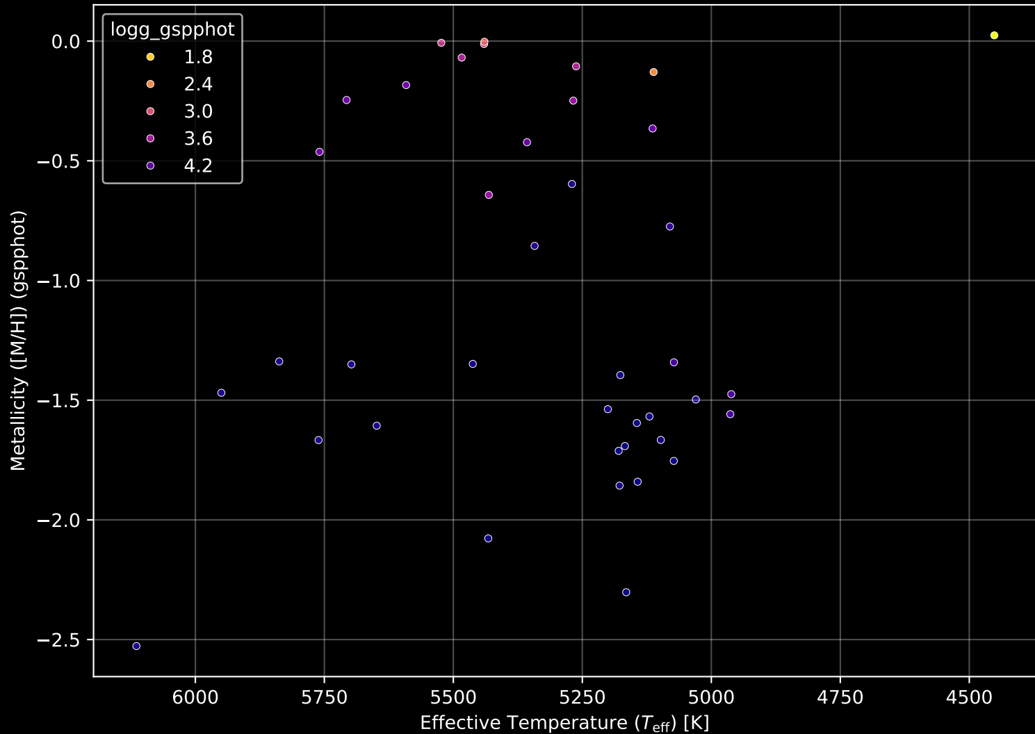
Gaia Stream: [NGC1851] Stellar Population Parameters (n= 40)
