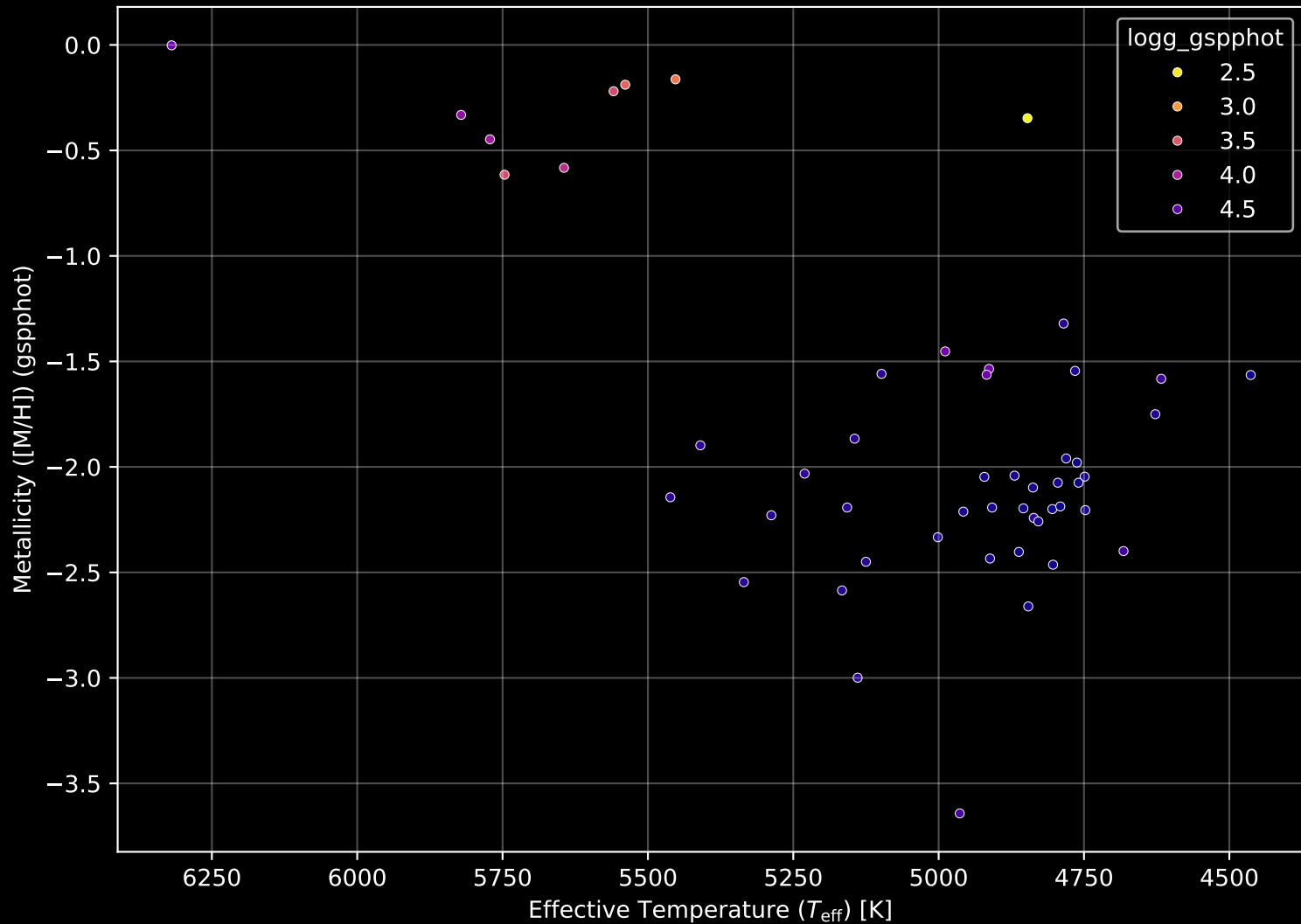
Gaia Stream: [NGC2808] Stellar Population Parameters (n= 51)
