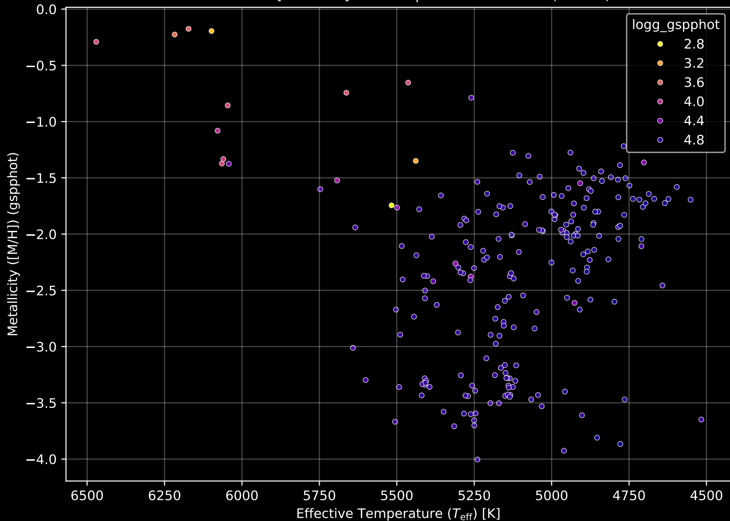
Gaia Stream: [NGC6101] Stellar Population Parameters (n= 218)
