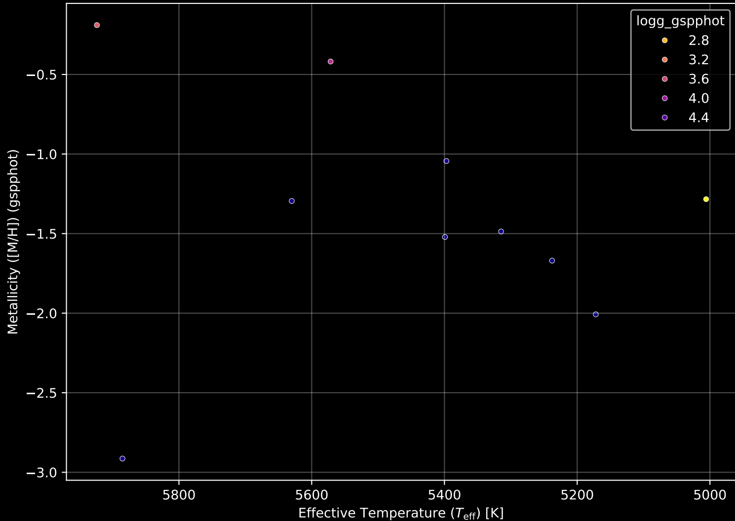
Gaia Stream: [NGC7089] Stellar Population Parameters (n= 10)
