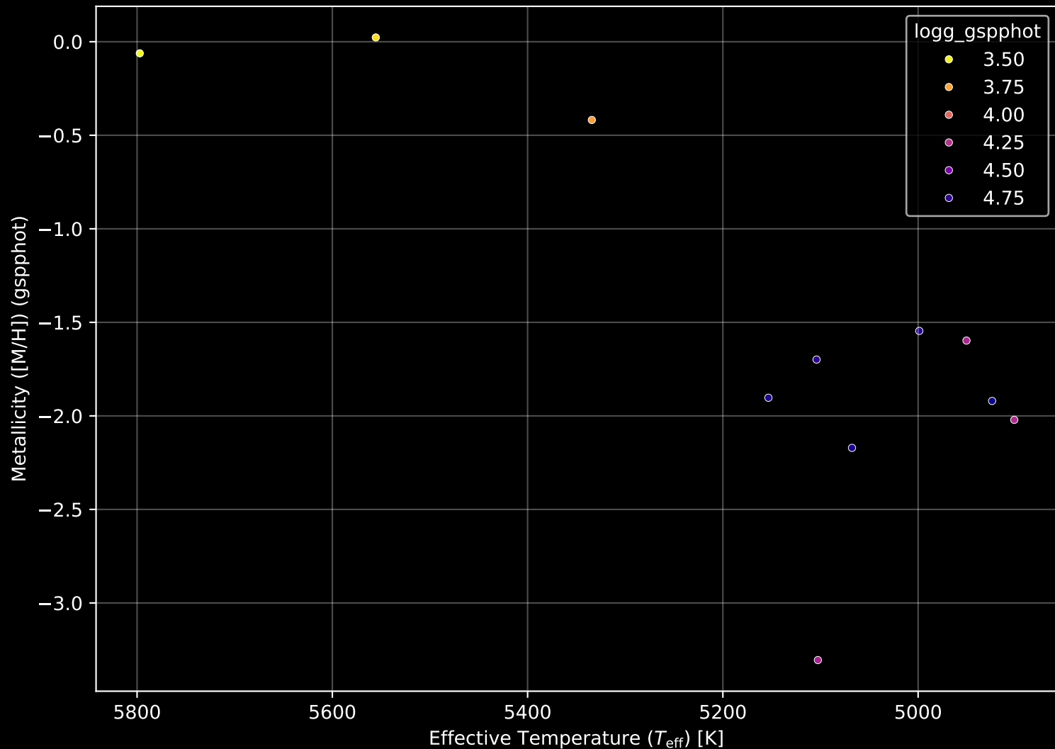
Gaia Stream: [NGC7492] Stellar Population Parameters (n= 11)
