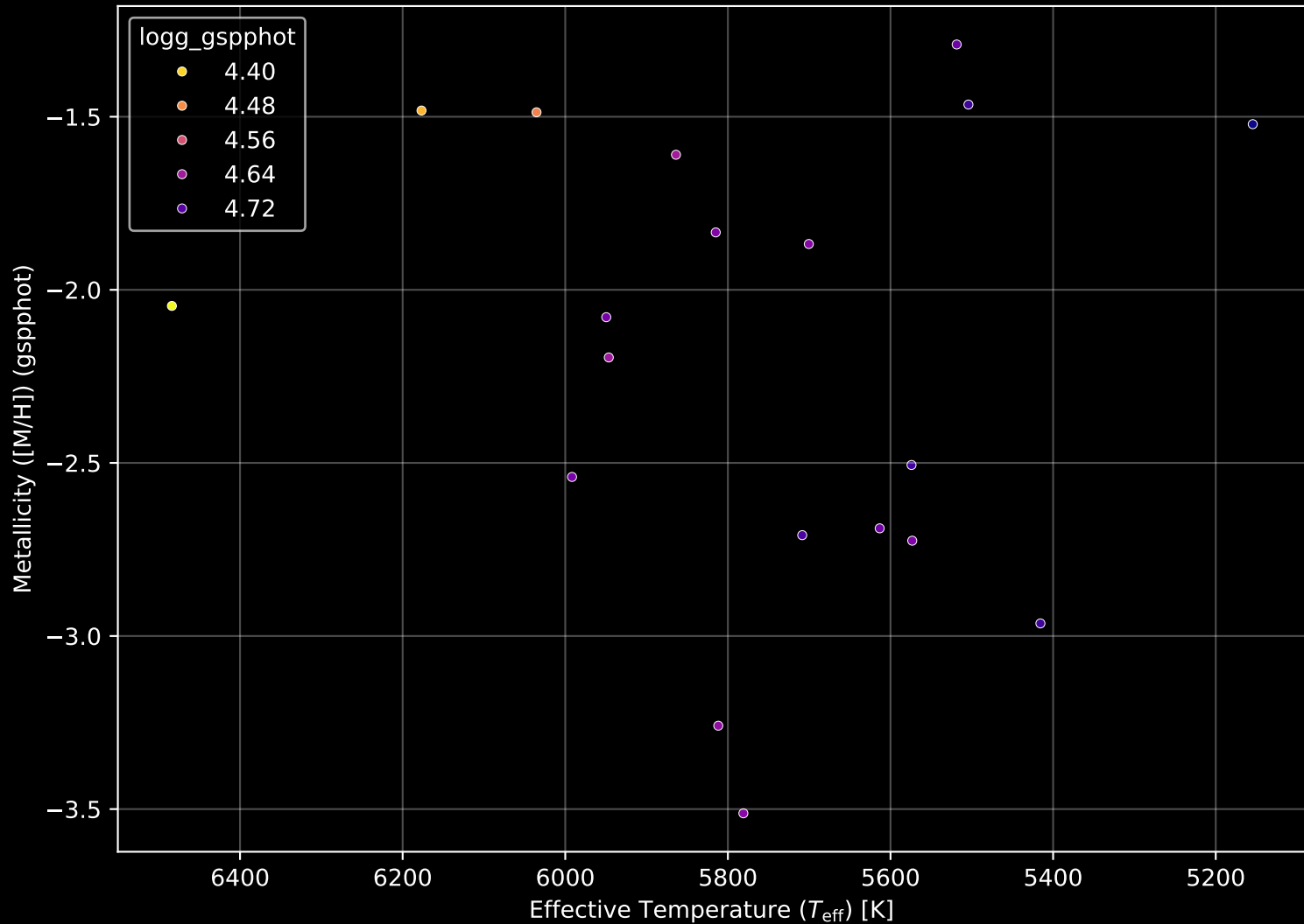
Gaia Stream: [New-16] Stellar Population Parameters (n= 19)
