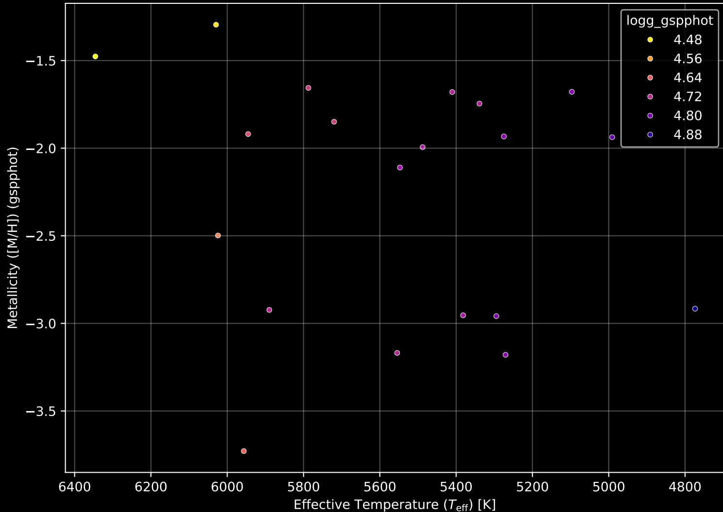
Gaia Stream: [New-23] Stellar Population Parameters (n= 20)
