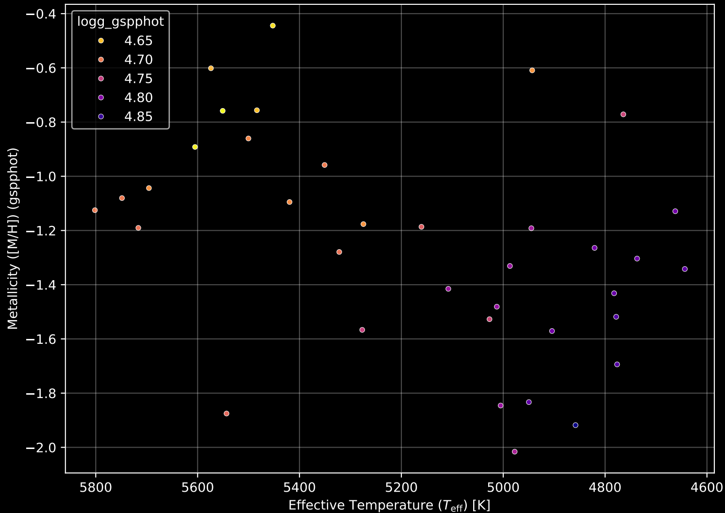
Gaia Stream: [New-24] Stellar Population Parameters (n= 36)
