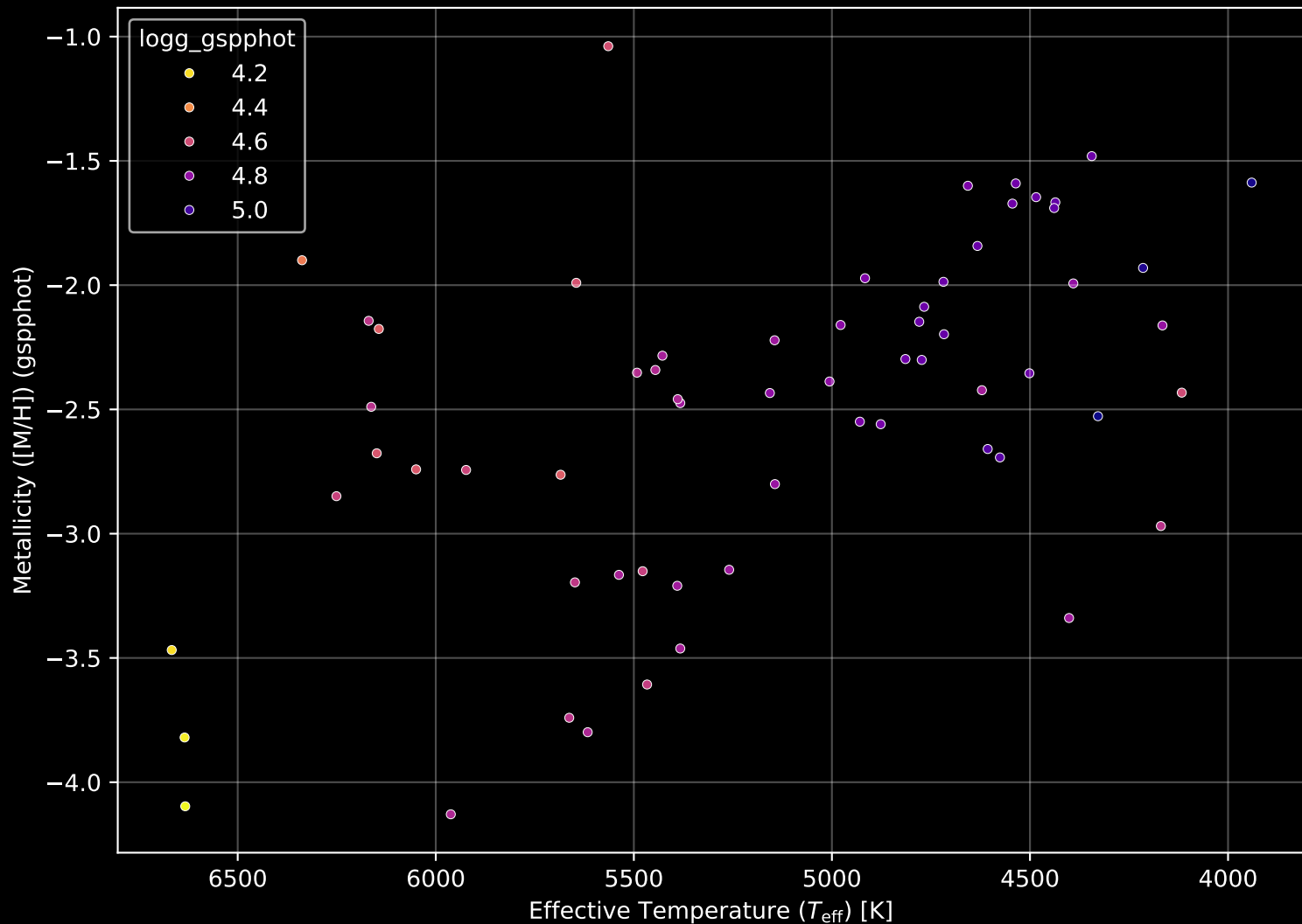
Gaia Stream: [New-3] Stellar Population Parameters (n= 63)
