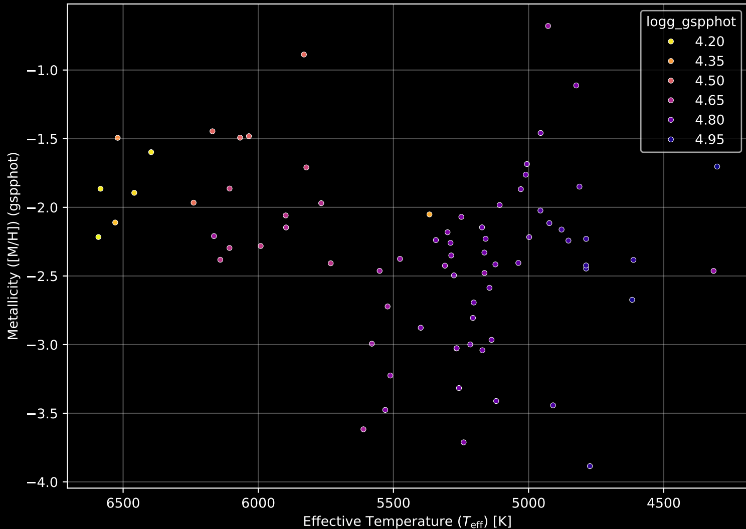
Gaia Stream: [New-6] Stellar Population Parameters (n= 76)
