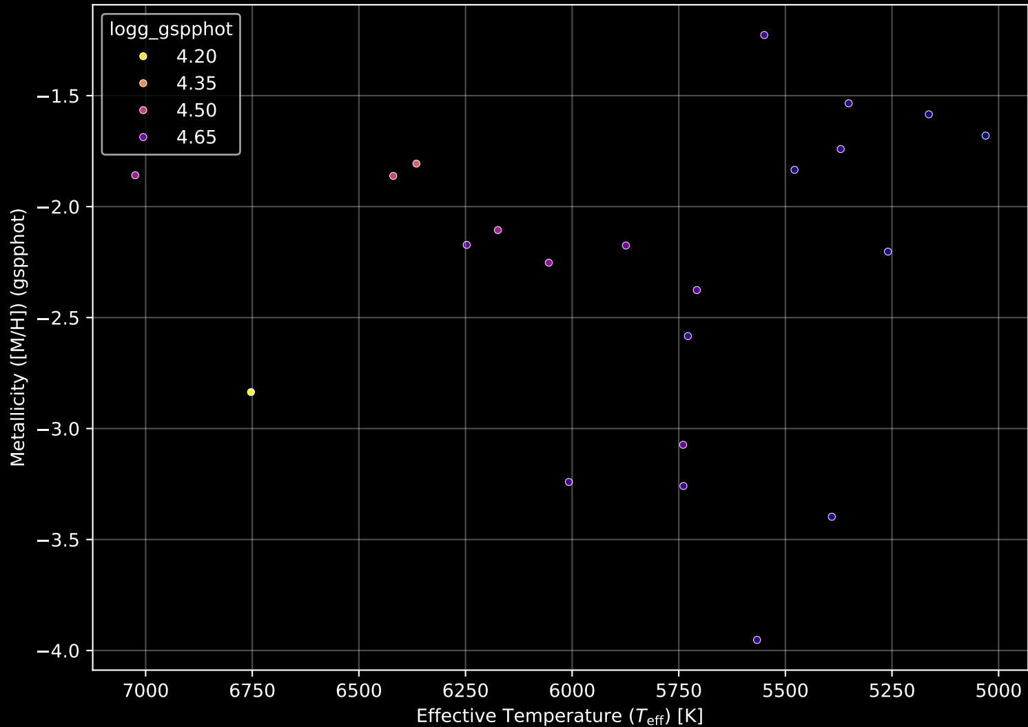
Gaia Stream: [New-7] Stellar Population Parameters (n= 22)
