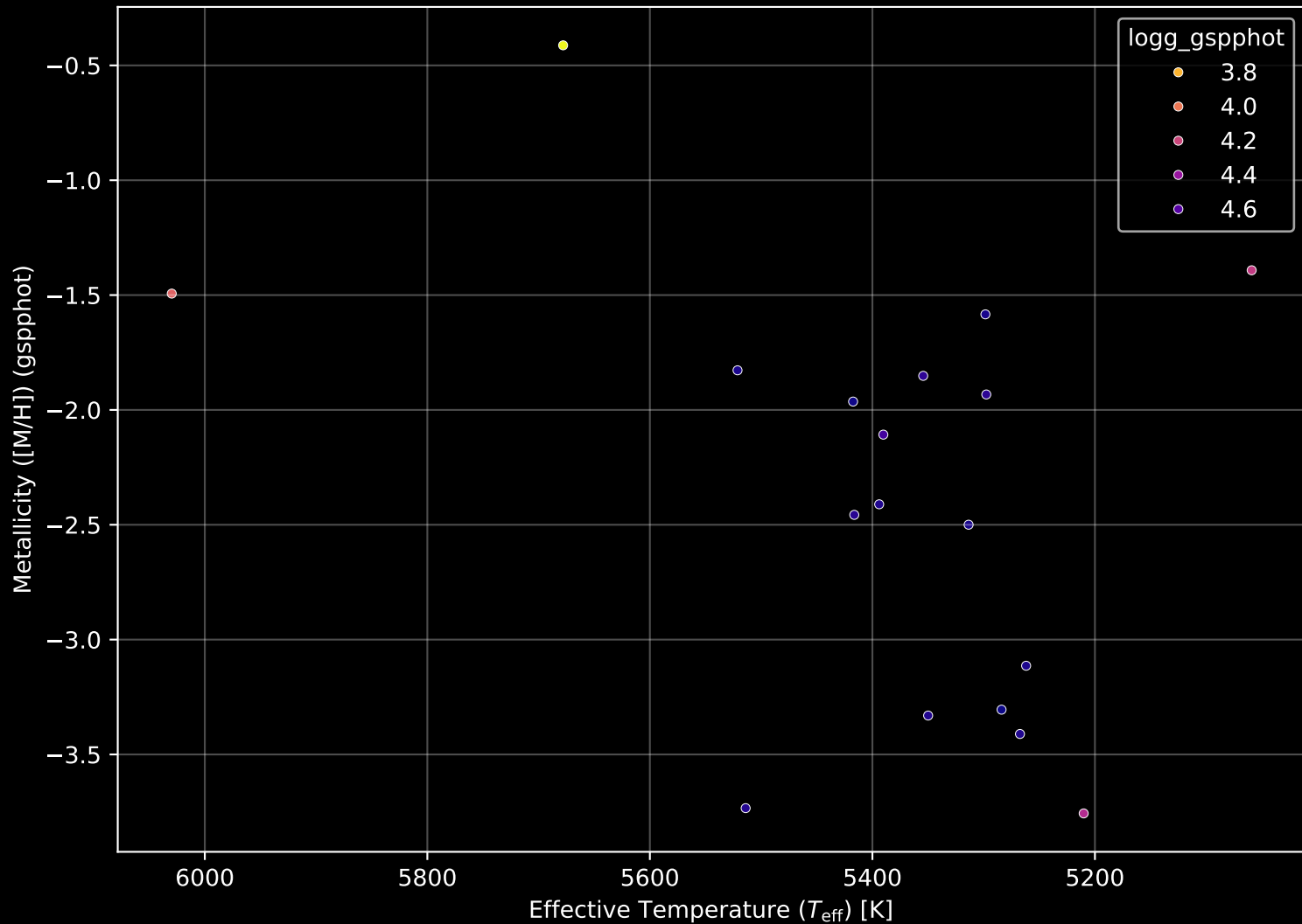
Gaia Stream: [Phoenix] Stellar Population Parameters (n= 18)
