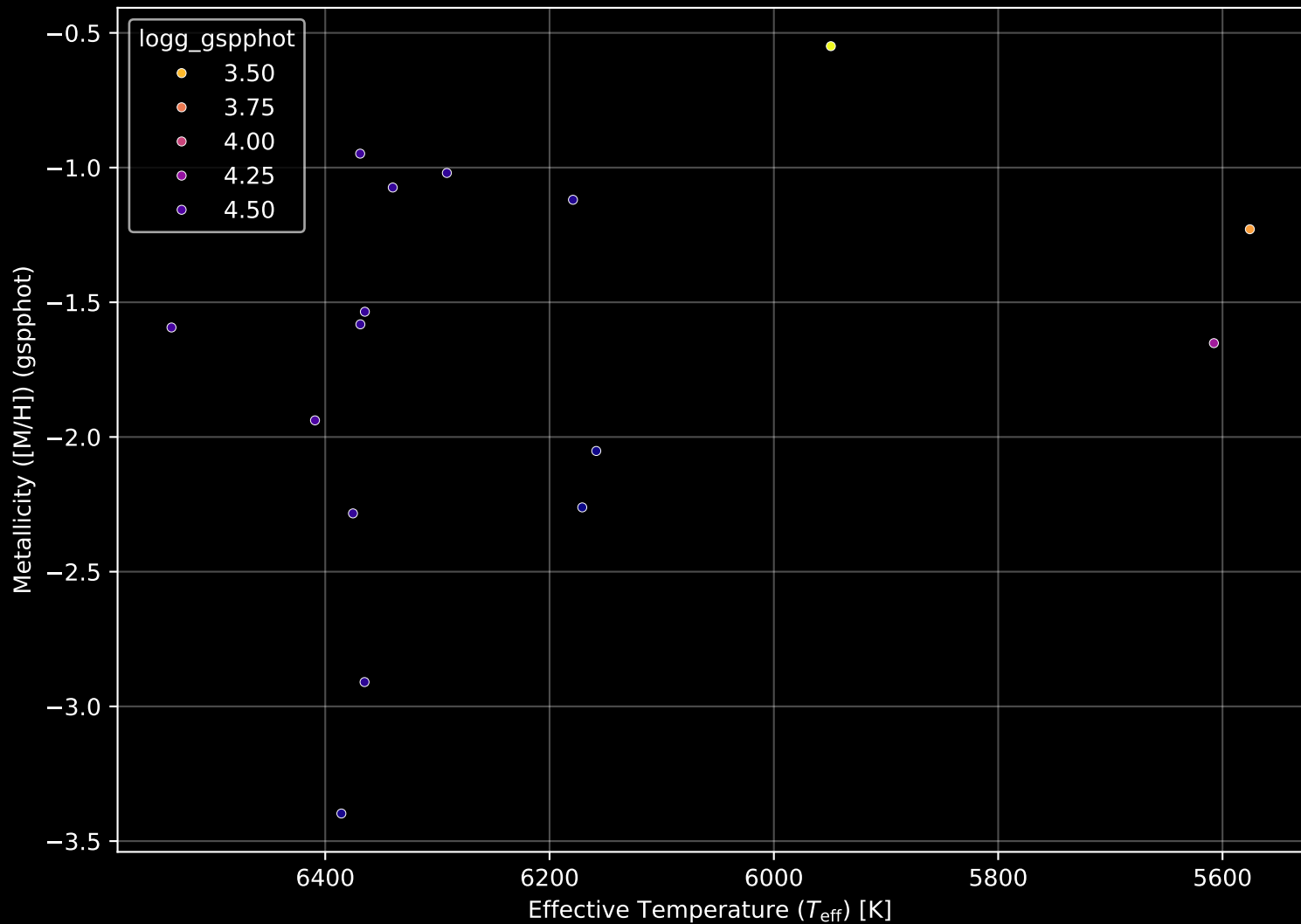
Gaia Stream: [SCP-S] Stellar Population Parameters (n= 16)
