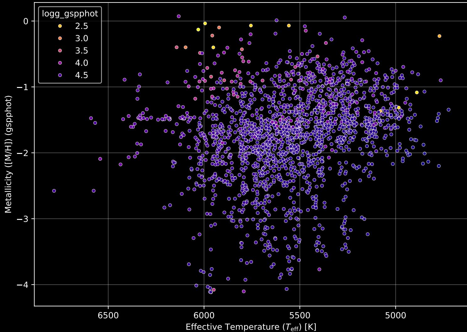
Gaia Stream: [Svol] Stellar Population Parameters (n= 1838)
