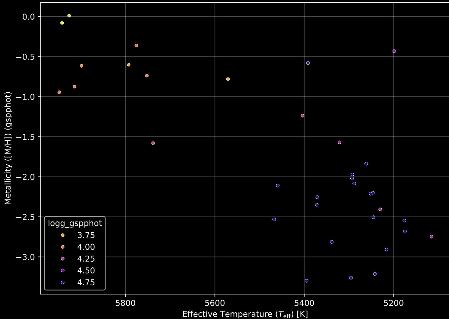
Gaia Stream: [Tuc-3] Stellar Population Parameters (n= 34)
