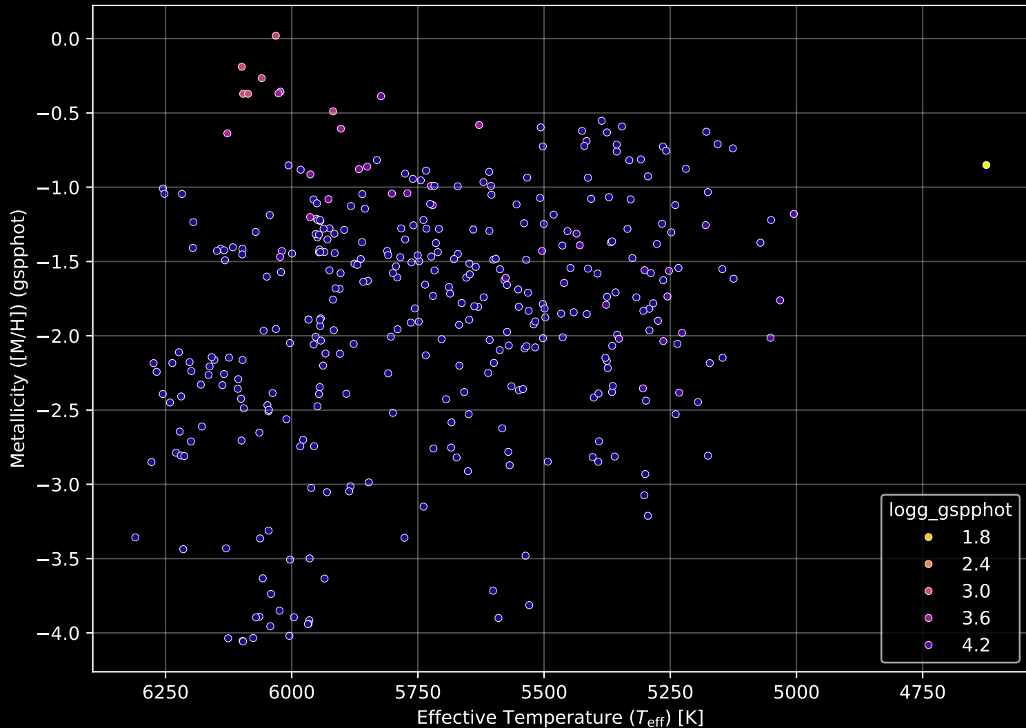
Gaia Stream: [Ylgr] Stellar Population Parameters (n= 371)
