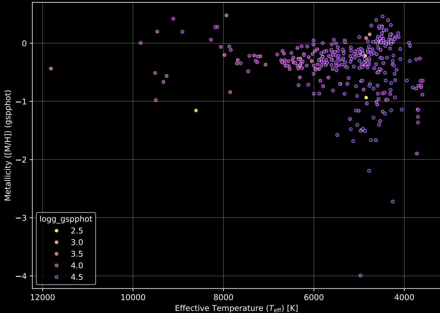
Gaia Cluster: [ASCC_111] Stellar Population Parameters (n= 329)
