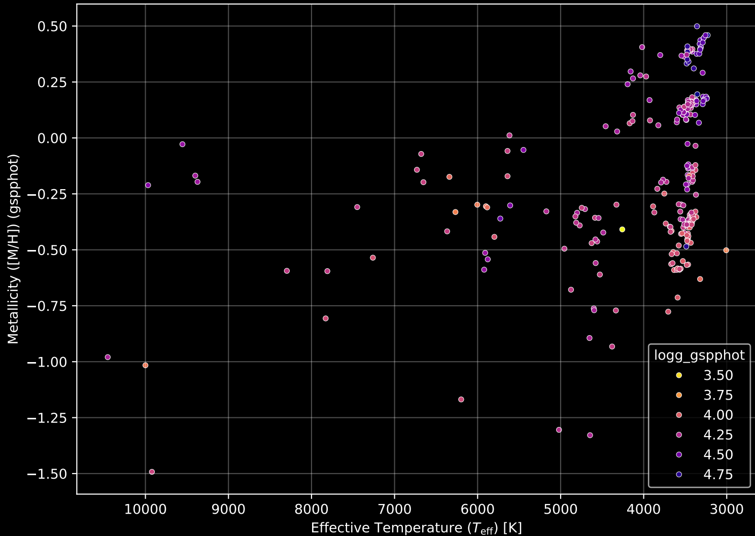
Gaia Cluster: [ASCC_16] Stellar Population Parameters (n= 276)
