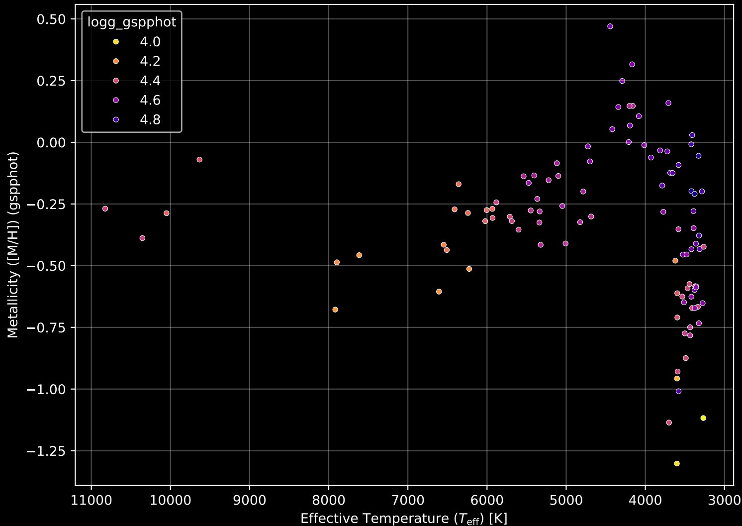
Gaia Cluster: [ASCC_41] Stellar Population Parameters (n= 103)
