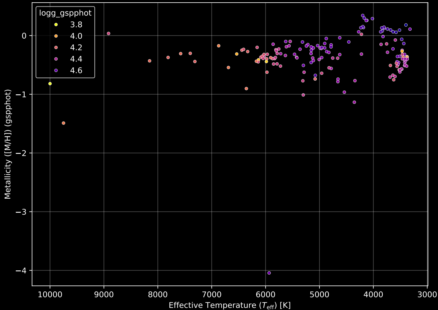
Gaia Cluster: [ASCC_58] Stellar Population Parameters (n= 161)
