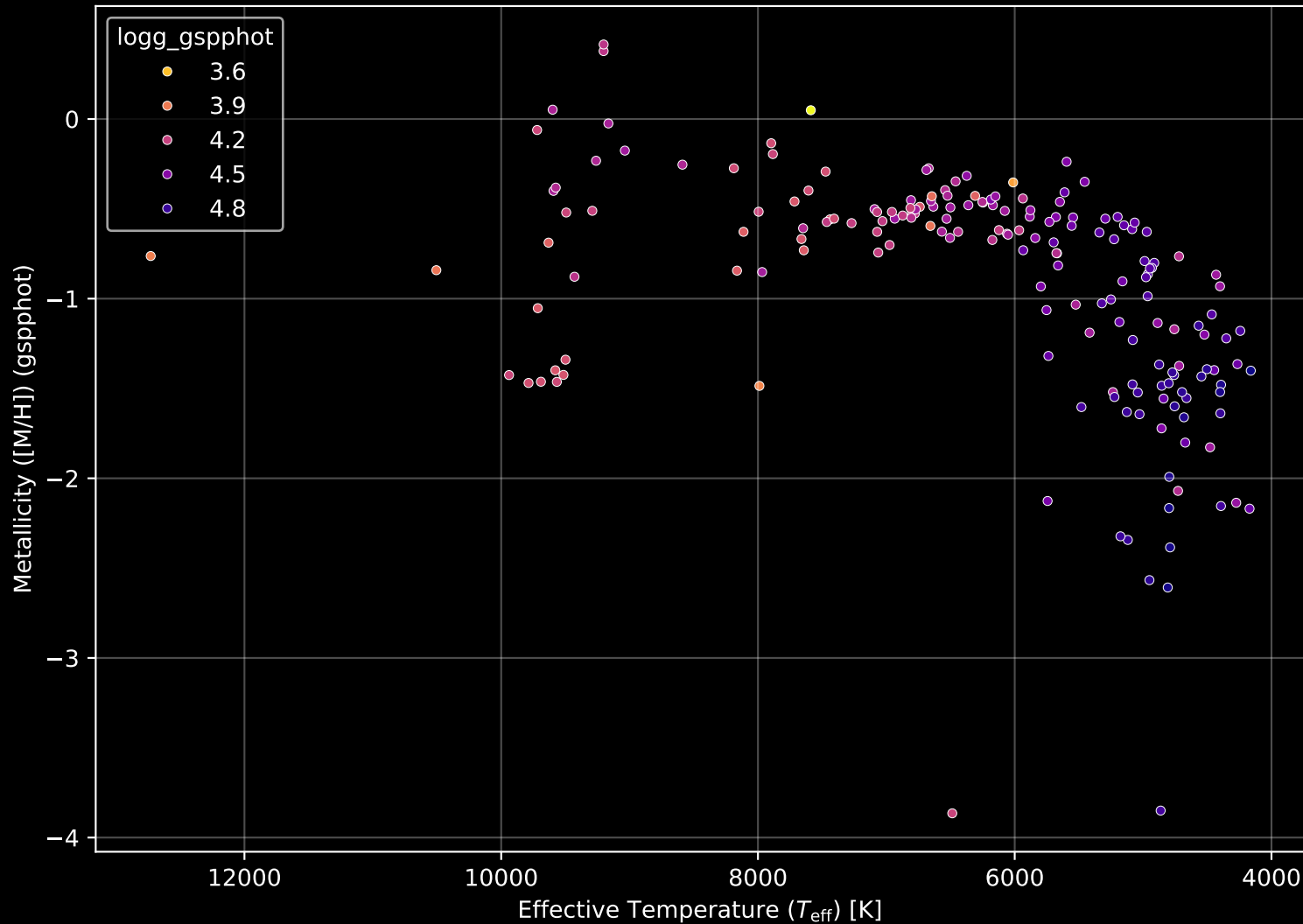
Gaia Cluster: [ASCC_6] Stellar Population Parameters (n= 183)
