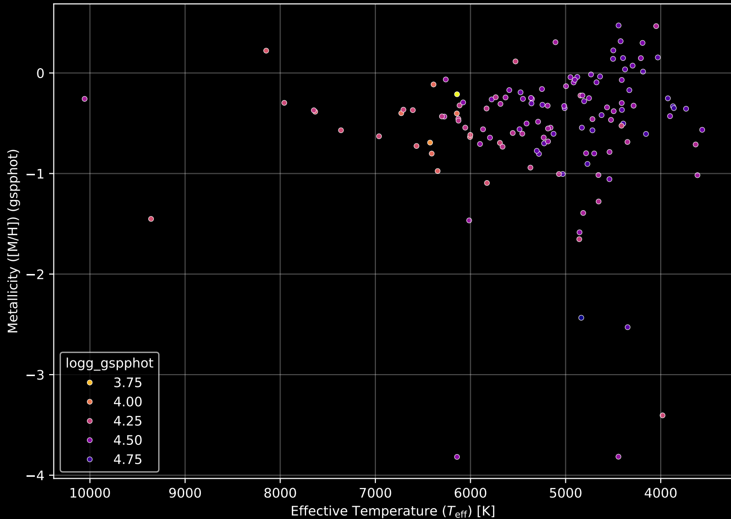
Gaia Cluster: [ASCC_73] Stellar Population Parameters (n= 132)
